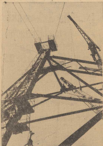
MONTAŻ wieży telewizyjnej w Leningradzie, której wysokość wynosić będzie 310 m. FOT — CAF
