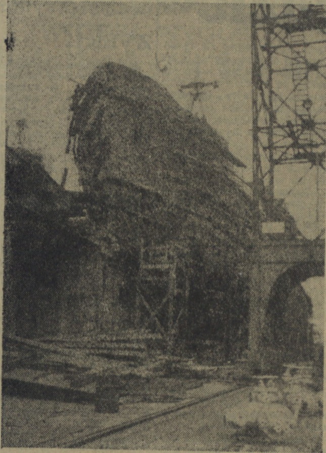
Stoczni szczyńska rozpoczęła produkcję w 1951 roku. Od tego czasu wodowano już 32 jednostki... Na zdjęciu: rudowłowiec B-32 na pochylni stożki.
