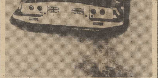
„PRINCESS ANNA” — największy na świecie poduszakowiec o długości 68,5 m — rozpocznie wkrótce regularne rejsy na kanale La Manche na trasie Dover—Boulogne—Calais. Zabierać będzie 416 pasażerów i 60 samochodów. Poduszakowiec ten, zaprojektowany w firmie brytyjskiej Cockerill, waży 300 ton i podczas podróży morskiej unosi się 4 metry nad powierzchnią wody. Rozpoczęcie rejsu planowane jest na 15 lipca. (Fot. CAF — CAMERA Press)
