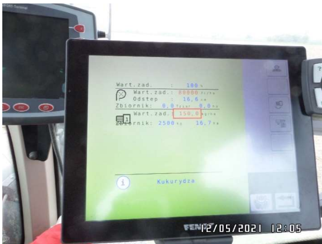
Rys. 3.5. Rzut GPS siewu i nawożenia rejestrowanego z ciągnika Fendt 828. Źródło: własna dokumentacja fotograficzna prowadzonego doświadczenia.
