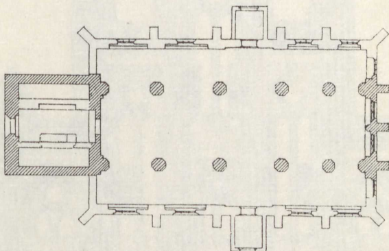
Fig. 40. Wollin; Nicolaikirche nach dem Umbau, Grundriss. 1:500.
