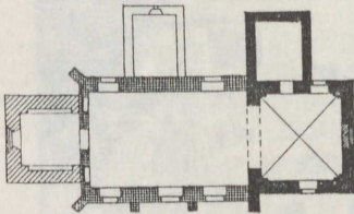
Fig. 14. Mellenthin; Kirche, Grundriss. 1:500.
