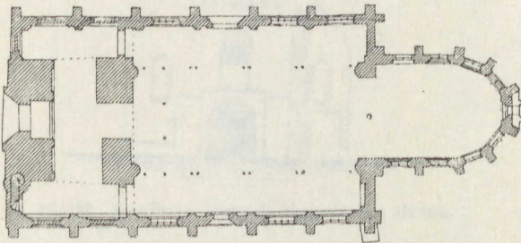
Fig. 30. Usedom; Marienkirche, vor dem Umbau. 1:500.
