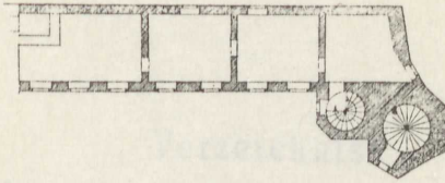
Fig. 46a. Ückermünde; Schloss, Grundriss. 1:500.
