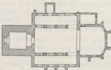
Fig. 7. Kolzow; Grundriss der früheren Kirche. 1 : 500.
