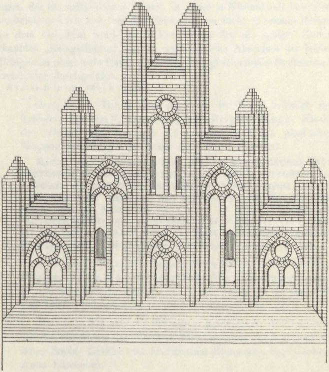
Fig. 43. Wollin; Nicolaikirche, Ostgiebel nach der Wiederherstellung. 1:200.
