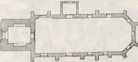
Fig. 38. Wollin; Georgenkirche, Grundriss vor dem Umbau. 1:500.
