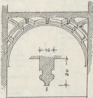
Fig. 46c. Ückermünde; Schloss, Querschnitt a—b.
