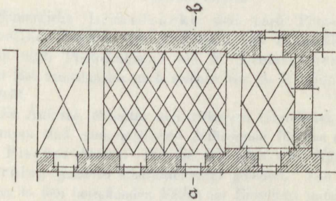
Fig. 46b. Ückermünde; Schloss, Gewölbbildung im Erdgeschoss. 1:200.
