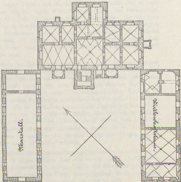
Fig. 19. Mellenthin; Schloss, Grundriss. 1:500.
