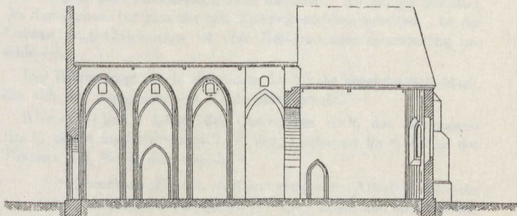
Fig. 8. Kolzow; ehemalige Kirche, Längsschnitt. 1 : 250.
