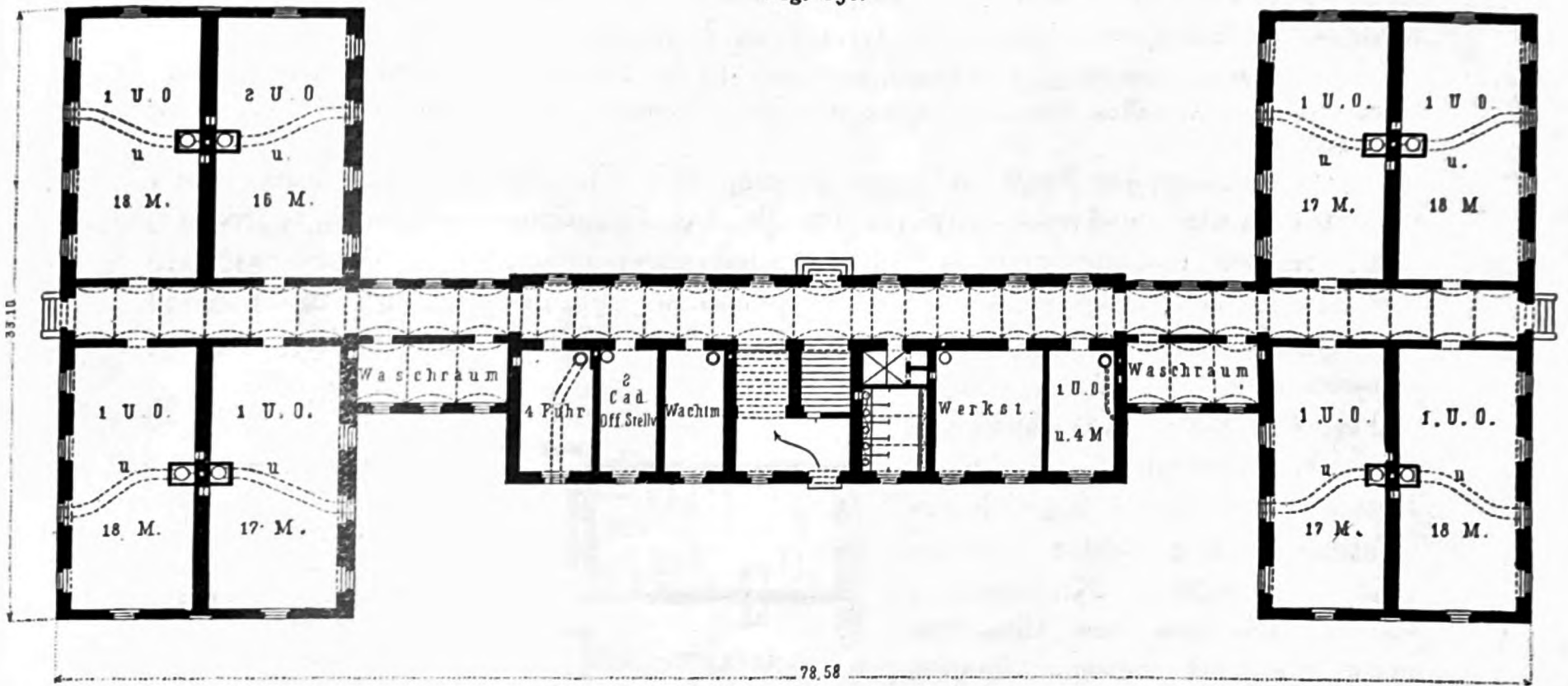
Mannschafts-Wohngebäude für 3 Eskadronen. — Erdgeschofs 142) .
