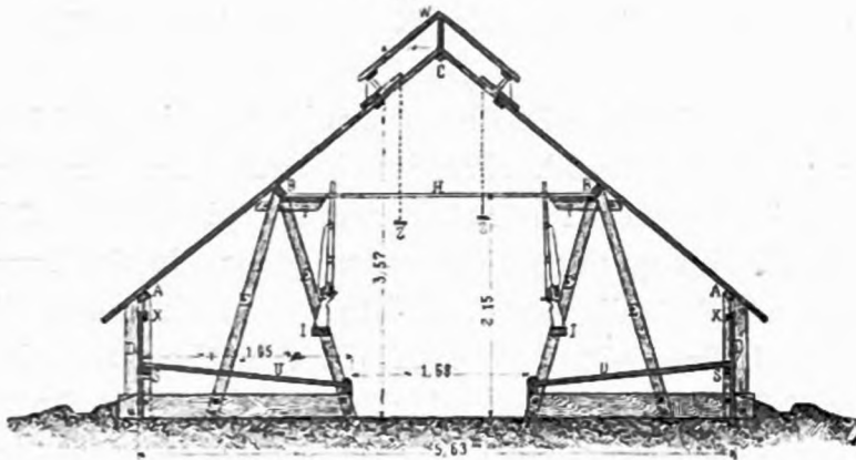
Querschnitt.
