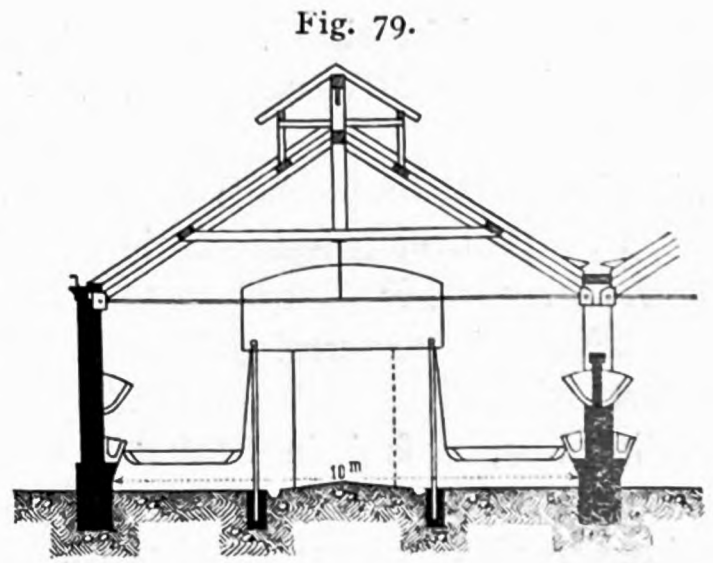
Stall für französische Kavalleriekasernen.
