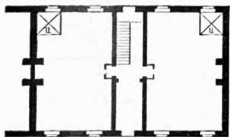
Infanteriekaserne zu Bury 120) .
