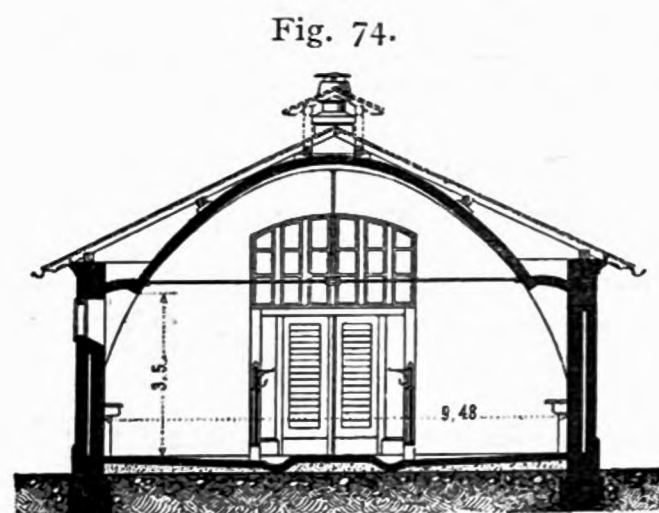
Stallsystem Gruber-Völckner .
