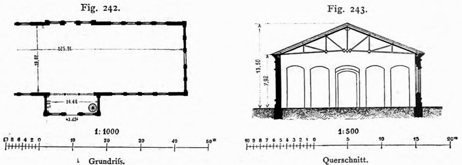
Exerzierhaus für 4 Bataillone zu Dresden.
