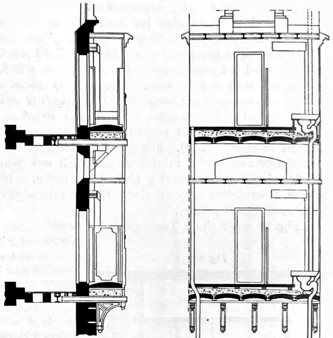
Schnitt nach a b.
