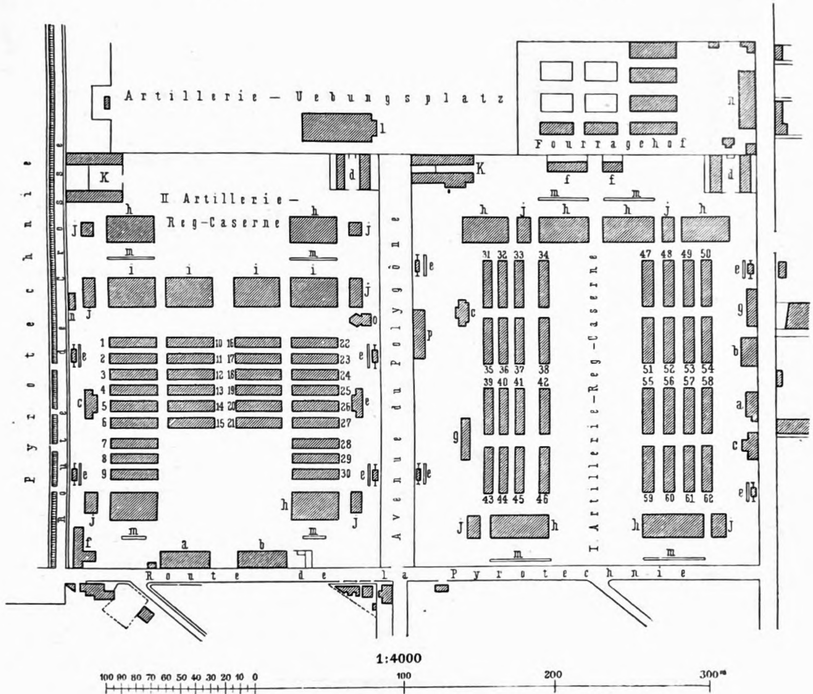
Artilleriekasernen zu Bourges.
