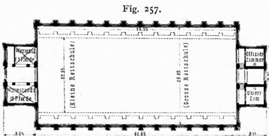
Große gedeckte Reitschule in Österreich-Ungarn 101) .
