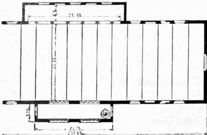
Grundriß.
