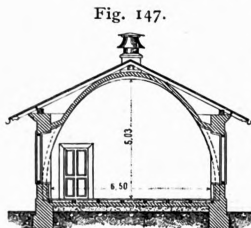
Pavillonkaserne. System Gruber-Völckner. \frac{1}{250} w. Gr.
