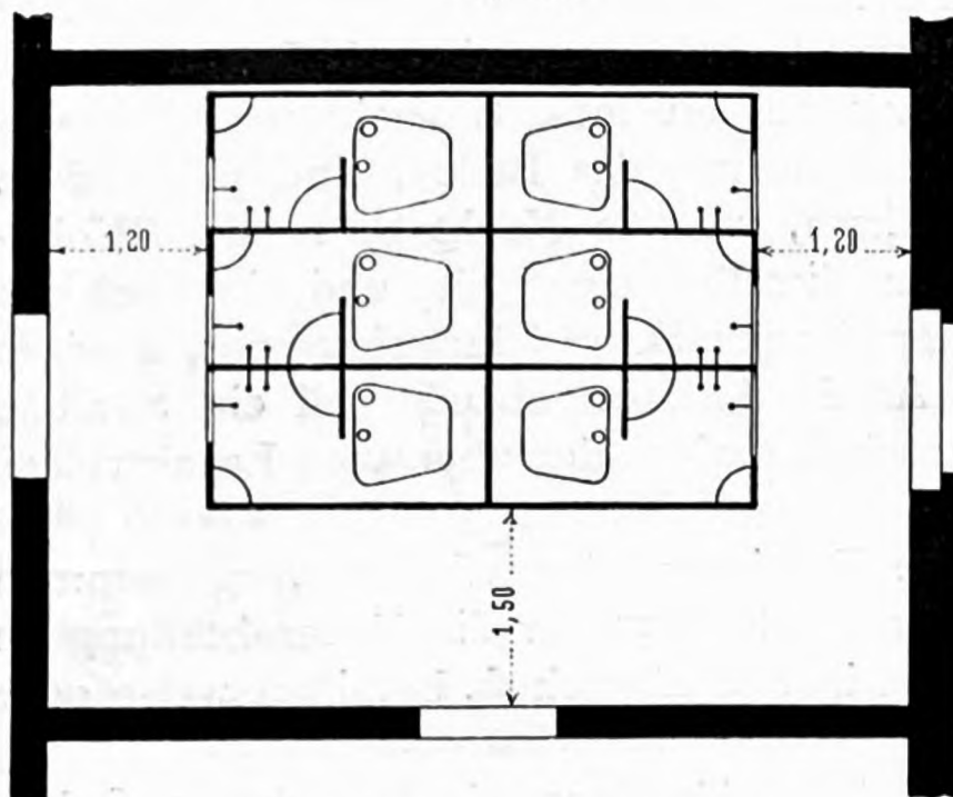
Gruppe von Brausebadzellen.
