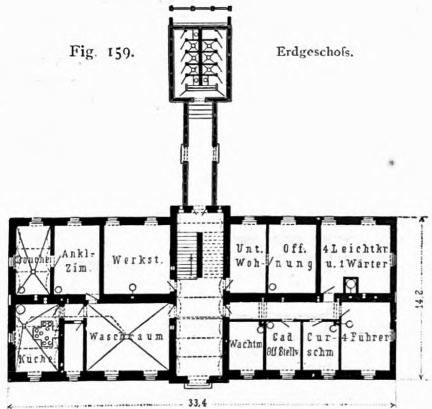
Osterreichische Eskadronkaserne 143) . — 1/500 w. Gr.
