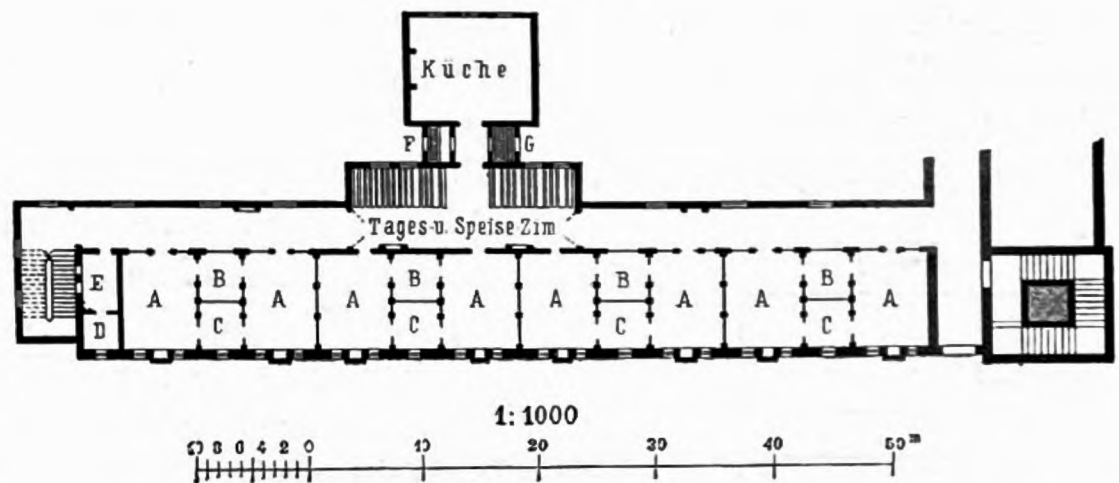
Morgan's Entwurf für das Kompagnierevier einer englischen Infanteriekaserne.
