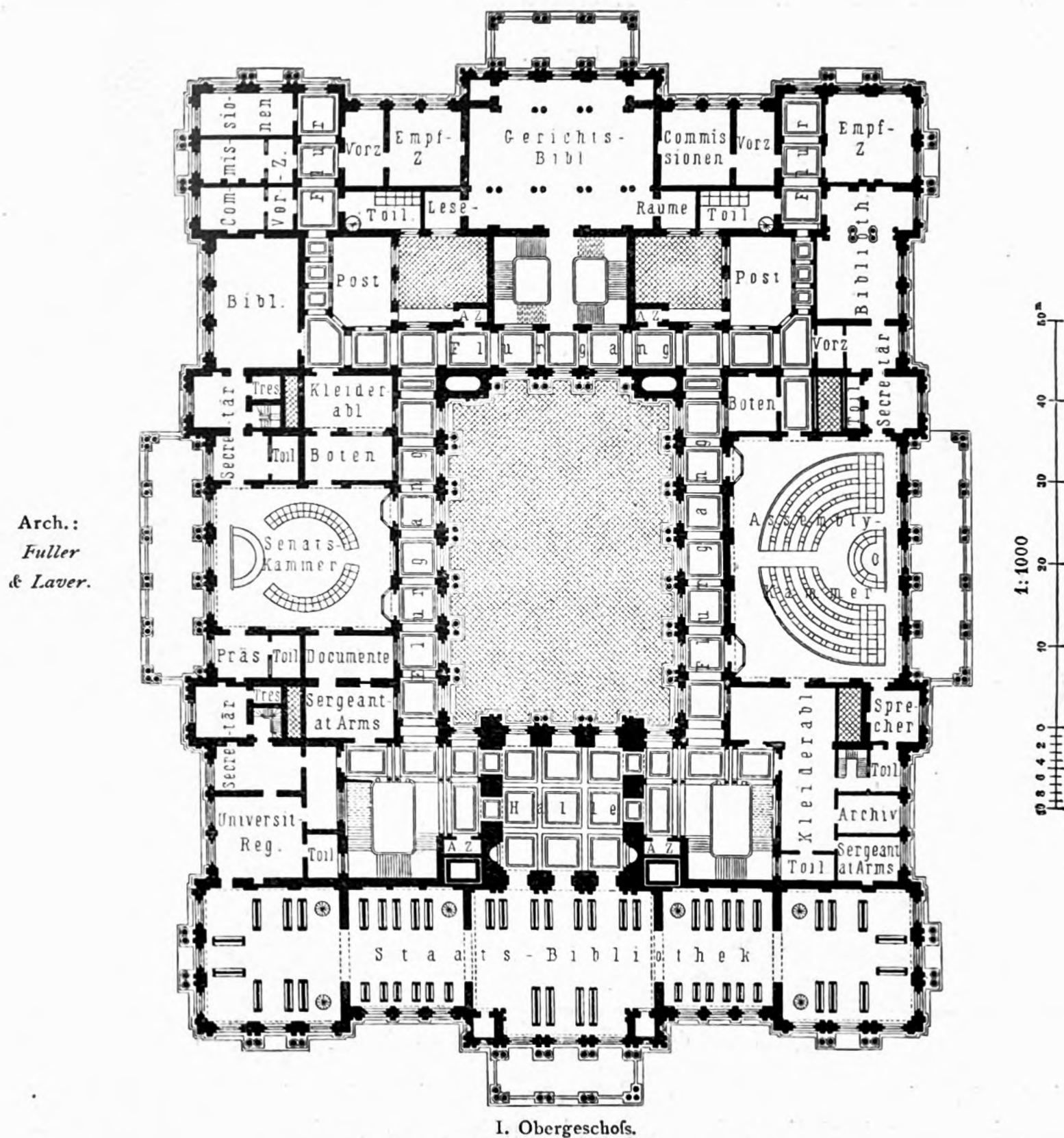
Kapitol für den Staat New-York zu Albany 52) .
