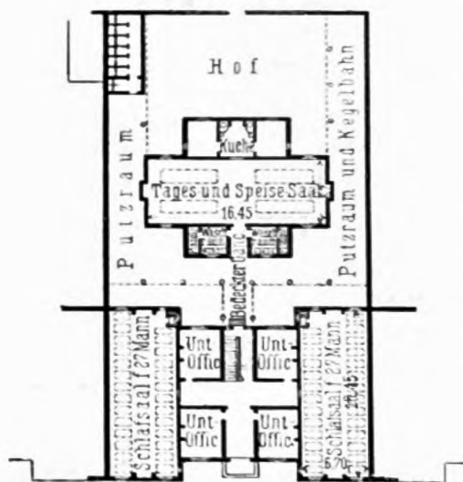
Guillaume's Entwurf für das Kompagniequartier einer englischen Infanteriekaserne.
