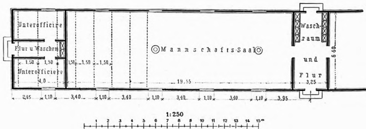
Tollet's Mannschaftspavillon.
