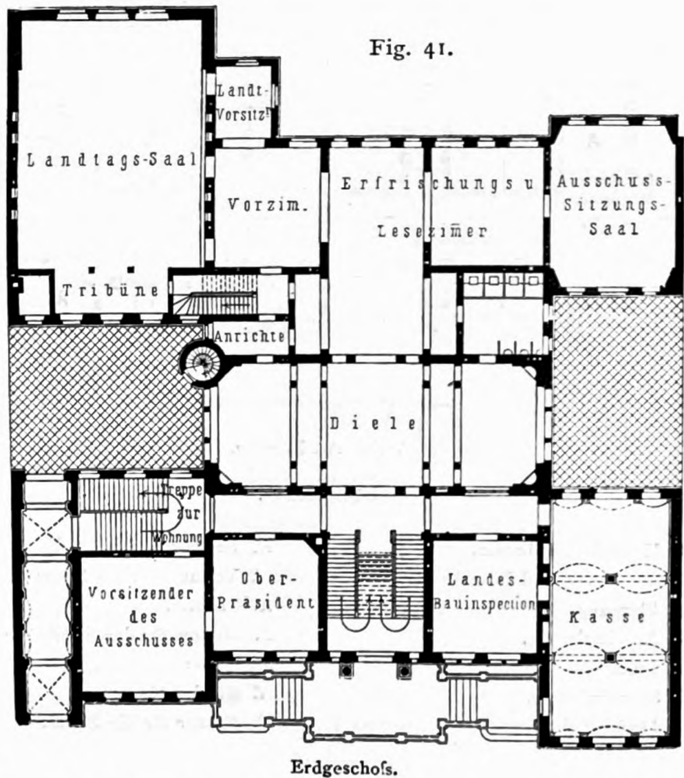
Landeshaus der Provinz Westpreußen zu Danzig 62) .
