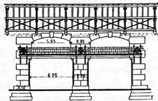
Teil des Längenschnittes.
