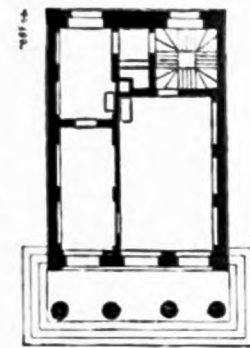
Ehemalige Wache am Potsdamer Thore zu Berlin 164 ).
