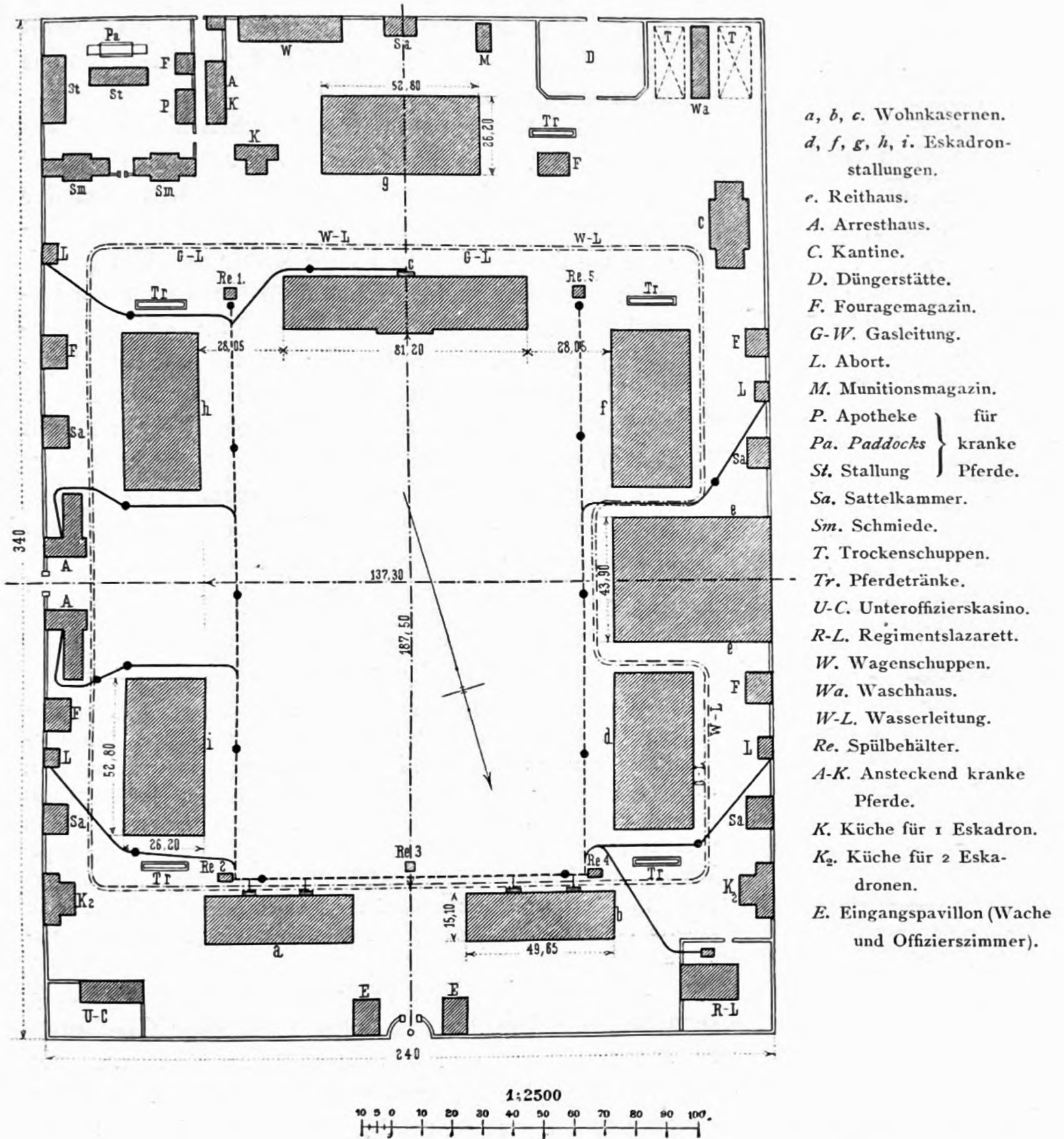
Kavallerieregiments-Kaserne zu Vincennes.
