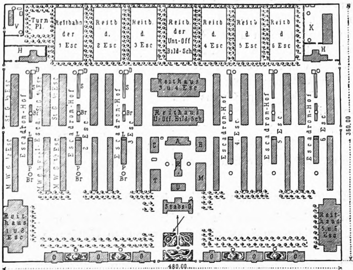
Österreichische Kavallerieregiments-Kaserne 113 ). — 1/5000 w. Gr. Pavillon-System Gruber-Völckner. Arch.: v. Gruber.
