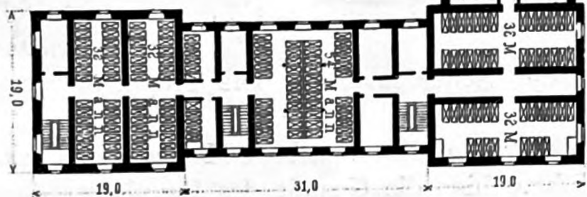
Fig. 105. I. Obergeschoss. 1/10000 w. Gr.
