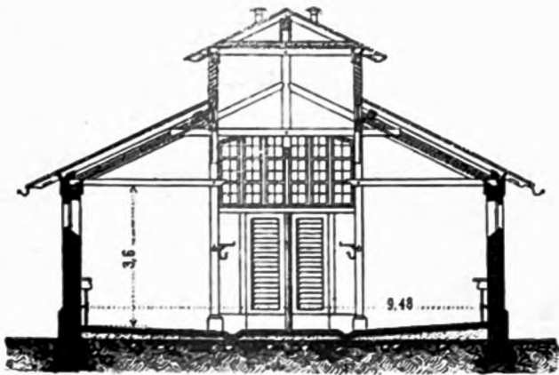
Österreichische Stallung älterer Konstruktion.
