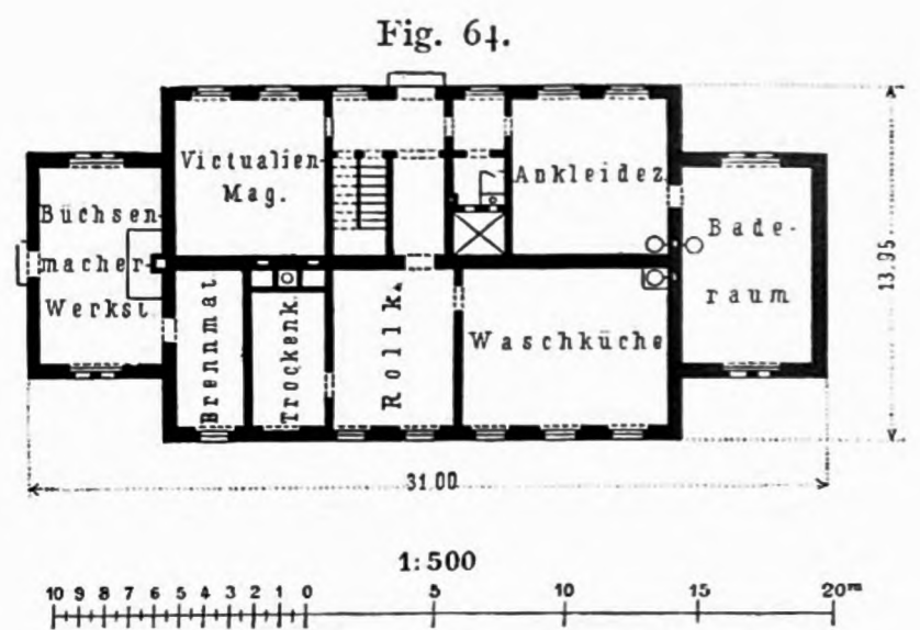
Bade- und Waschküchengebäude einer österreichischen Infanteriekaserne 107) , Arch.: v. Gruber.
