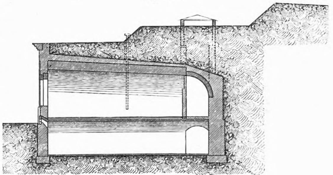
Querschnitt. — \frac{1}{250} w. Gr.
