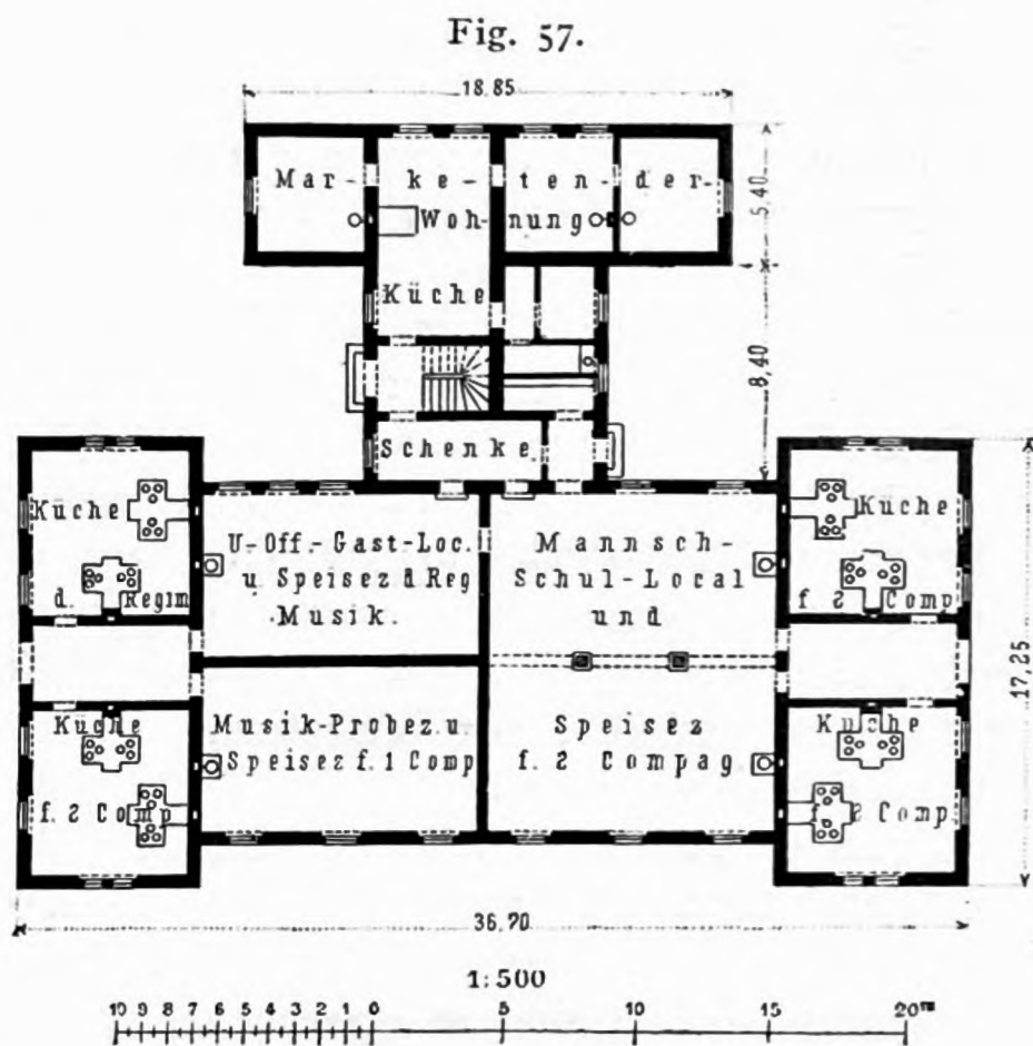
Marketenderei- und Küchengebäude einer österreichischen Regimentskaserne 101) .
