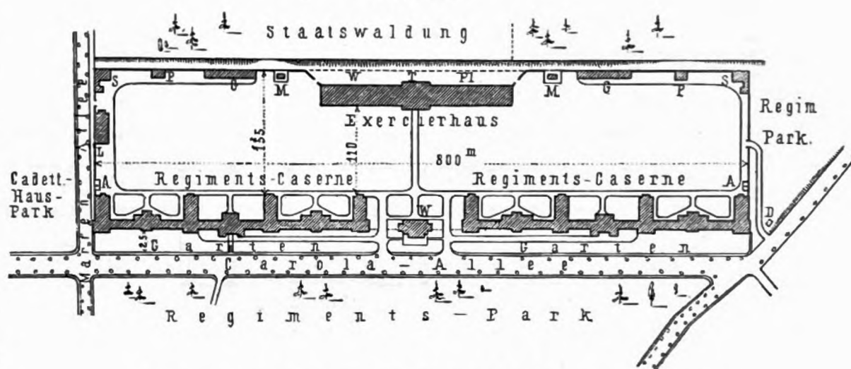
Kasernement für eine Infanteriebrigade zu Dresden.
