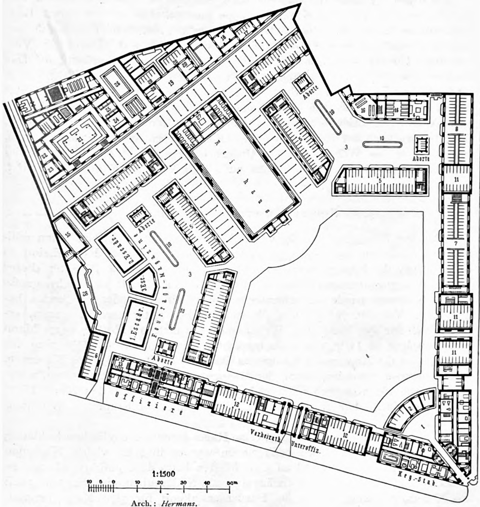
Preisgekrönter Entwurf zu einer Kaserne für 3 Eskadronen republikanischer Garde.
