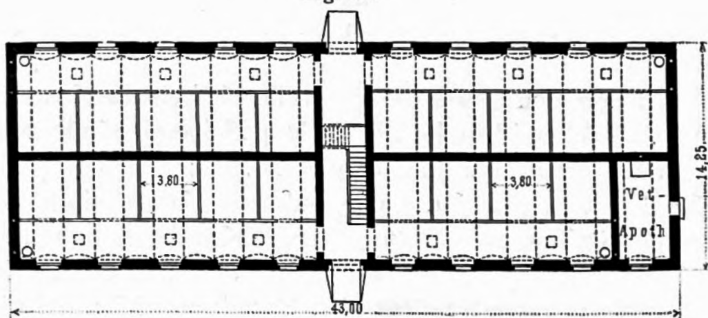
Krankenstall für ein österreichisches Kavallerieregiment 121) .
