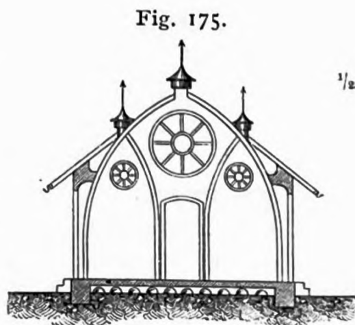
Querschnitt zu Fig. 173 u. 174.
