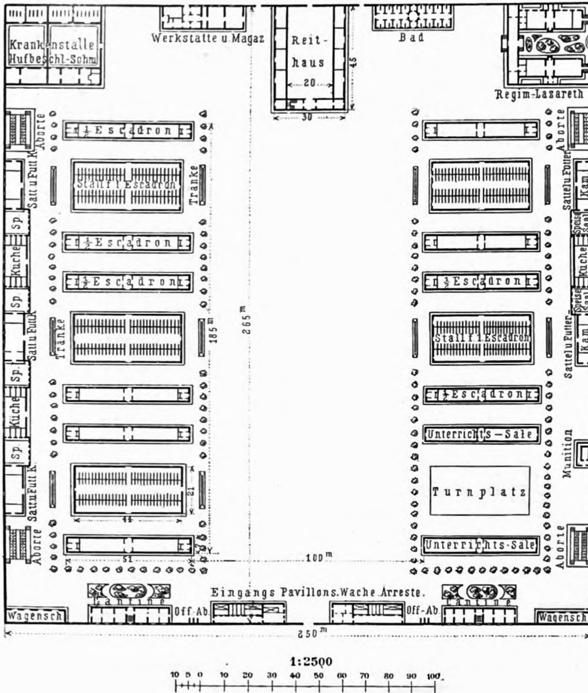
Tollet's Kaserne für ein Kavallerieregiment.
