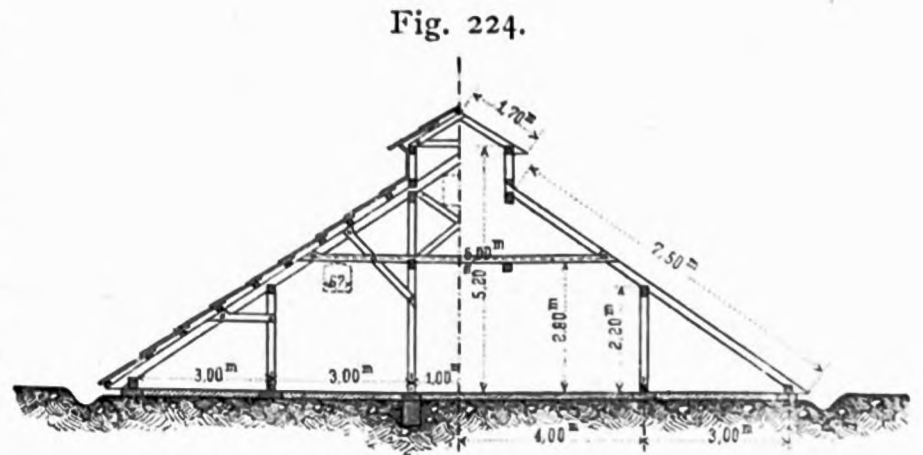
Hölzerne Stallbaracke. — \frac{1}{250} w. Gr.
