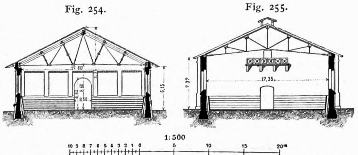
Normalplan eines preussischen Reithauses 160) .
