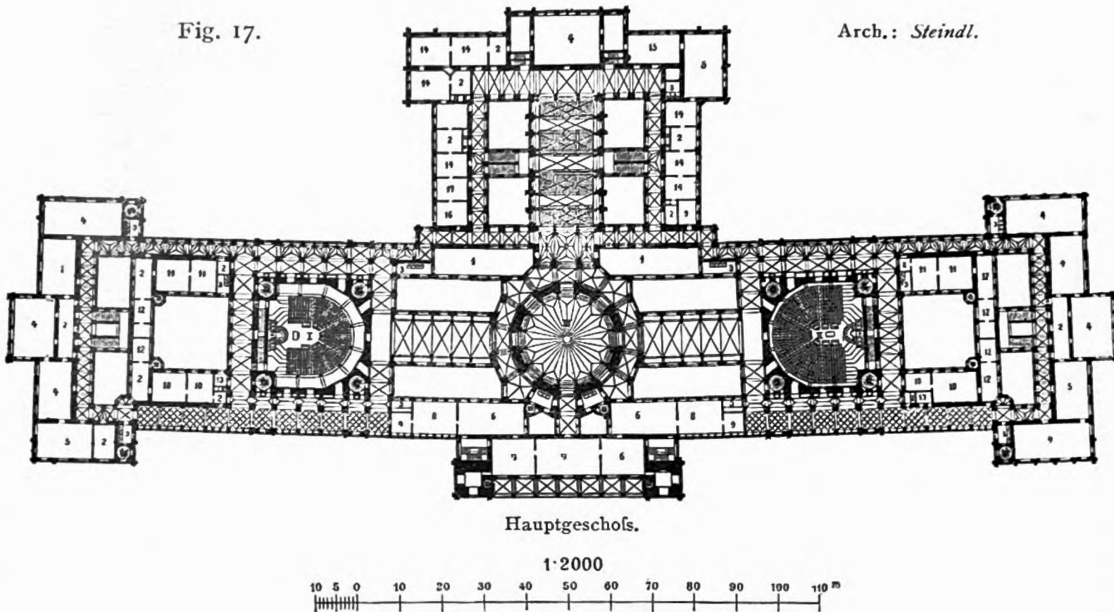
Parlamentshaus zu Budapest 51) .
