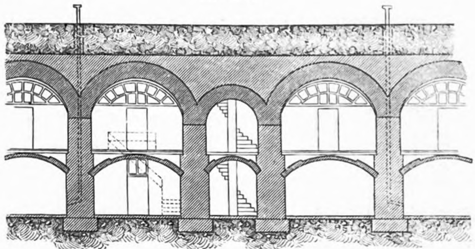
Längenschnitt. — \frac{1}{250} w. Gr.
