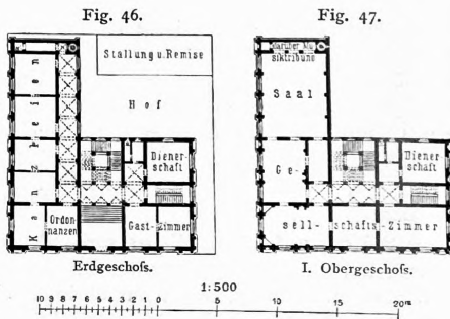
Entwurf für ein General-Kommando-Gebäude zu Stuttgart 86) . Arch.: Dollinger .
