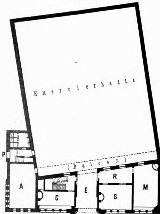
Hauptquartier des 2. Manchester-Freiwilligenregiments zu Manchester.
