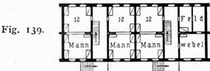
System der Militärquartierhäuser (Bataillonskasernen) zu Schwerin.
