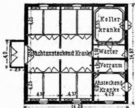
Krankenstall für ein Feldartillerieregiment zu Dresden.
