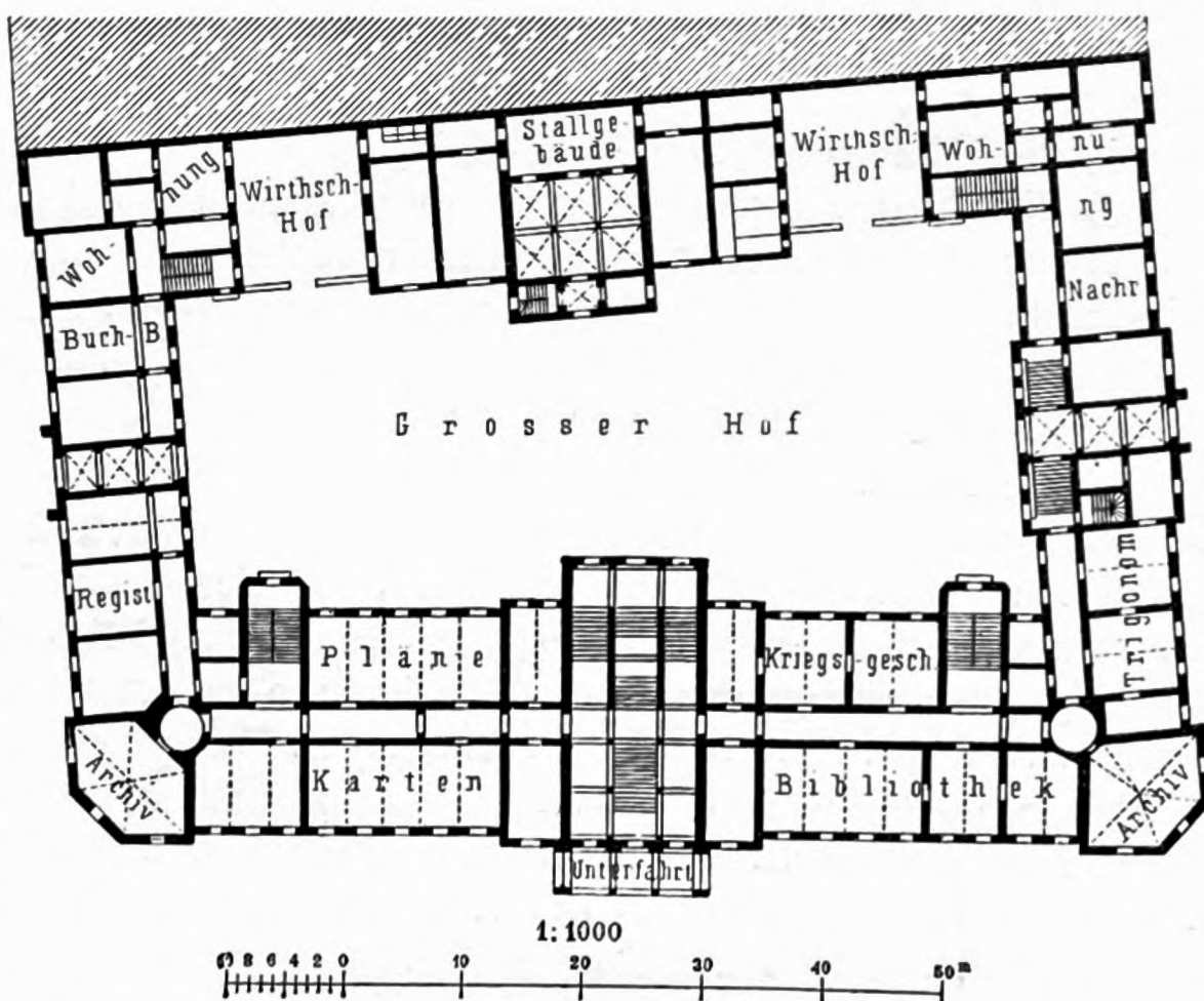
Generalstabs-Gebäude zu Berlin. — Ursprüngliche Anlage 87) . Arch.: Goedeking .
