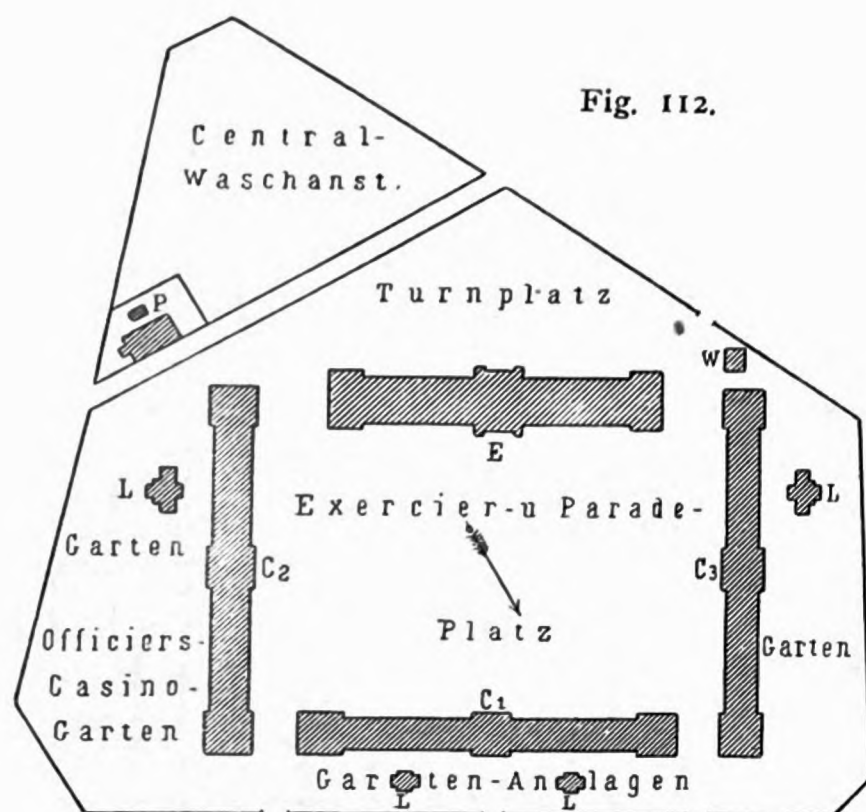
Kasernement des Kaiser-Franz-Garde-Grenadierregiments zu Berlin 134) . — 1/5000 w. Gr.
