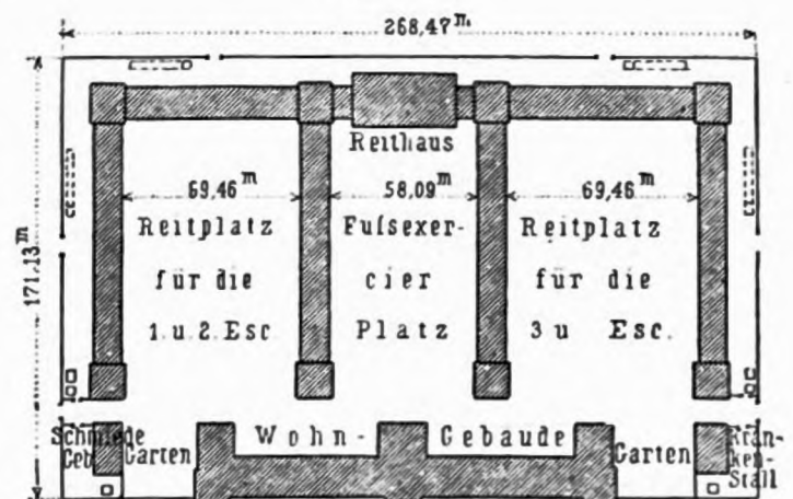
Kaserne für das 2. Garde-Ulanenregiment zu Moabit 135) . — \frac{1}{5000} w. Gr.
