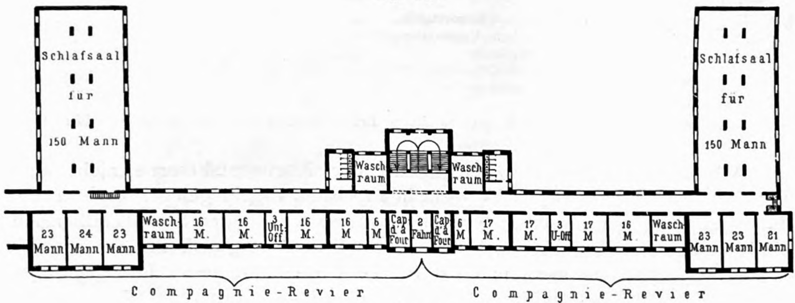
Linker Flügel (III. Obergeschoss).
