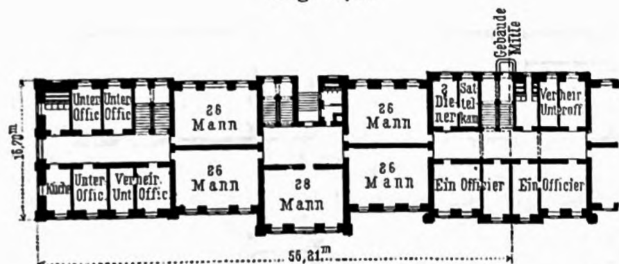
Kaserne für 2 Eskadronen Kavallerie zu Oschatz.
