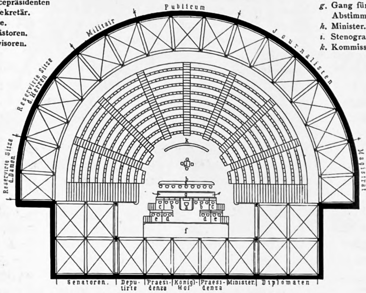
Sitzungssaal des Abgeordnetenhauses zu Rom 24) .
