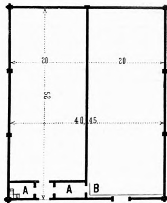
Französisches Reithaus.
