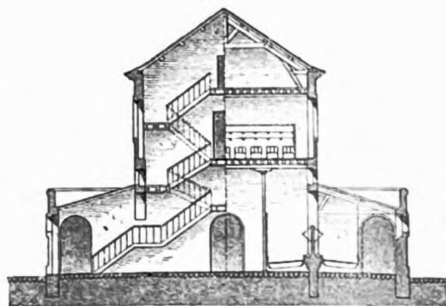
Querschnitt nach CD. — 1/500 w. Gr.
