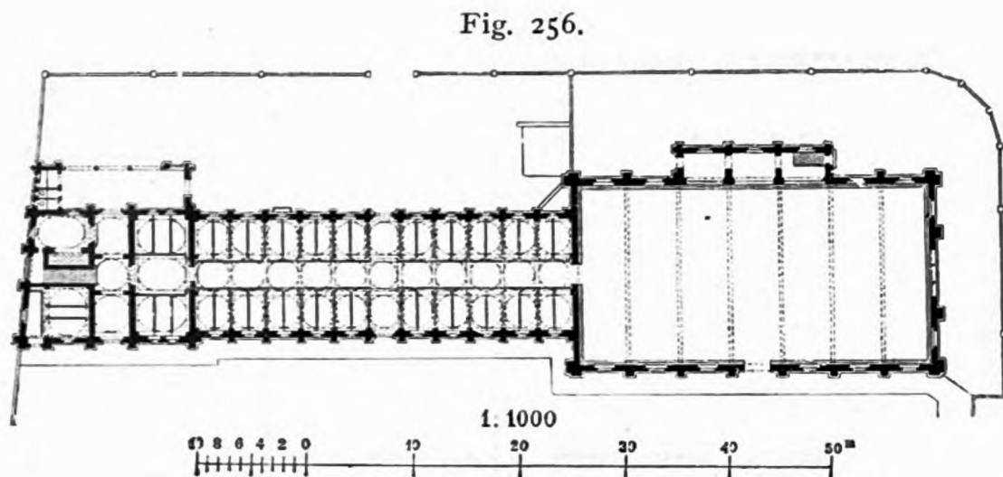
[Reithaus und Stallungen der Kriegsschule zu Kassel.
