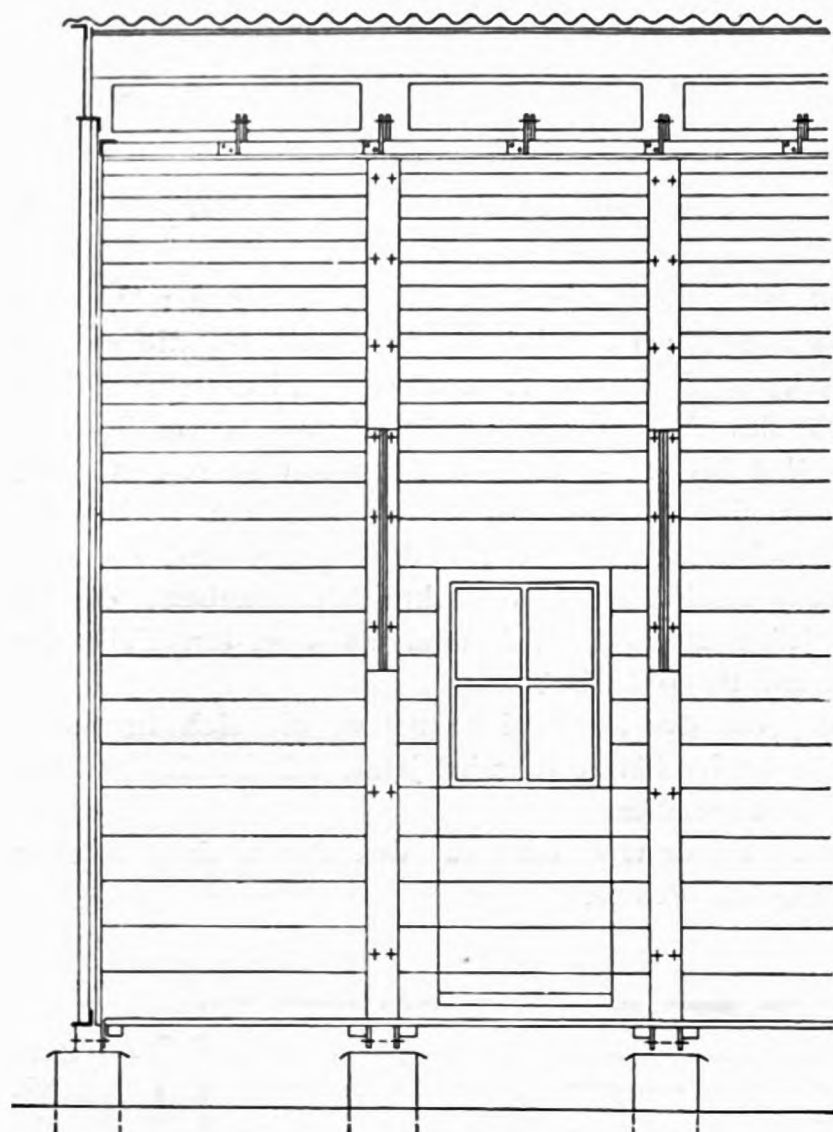
Längenschnitt. — \frac{1}{50} w. Gr.
