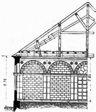
Exerzierhaus bei Berlin 157) .
