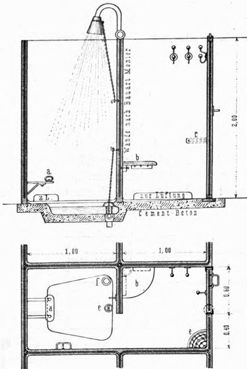
Brausebad von Knoblauch.
