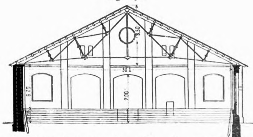
Querschnitt zu Fig. 258. — \frac{1}{500} w. Gr.
