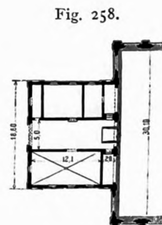
Reitschule der Kaserne zu Oedenburg.
