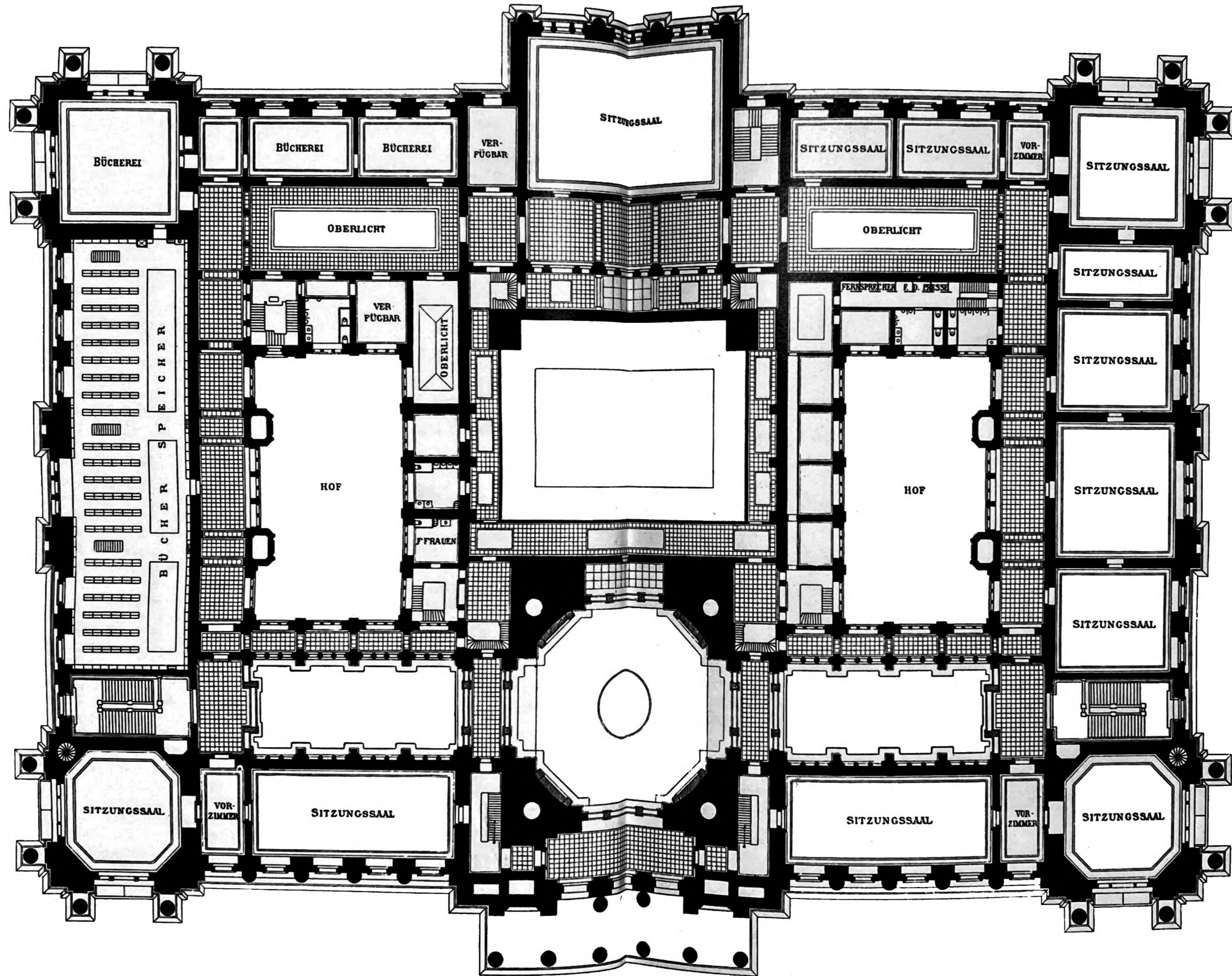
Deutsches Reichstagsgebäude zu Berlin.
