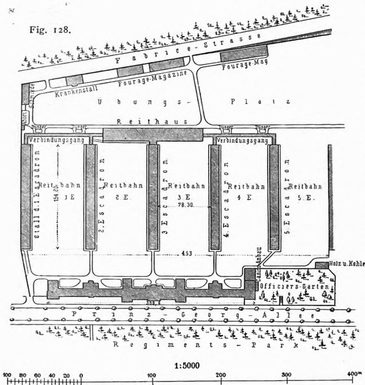
Kasernement für ein Regiment Kavallerie zu Dresden.
