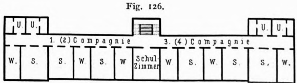
System der althannoverschen Kasernen (I. u. II. Obergeschos).
