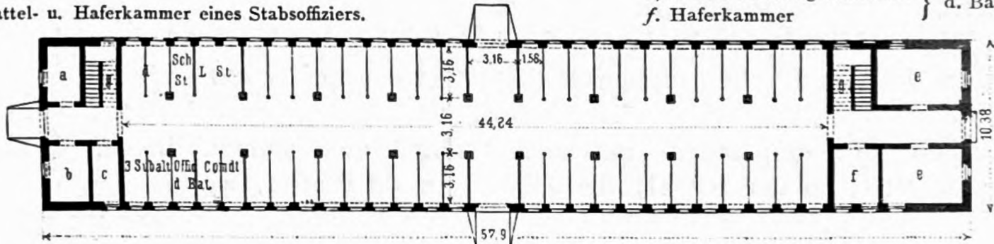
Österreichische Batteriestallung 119) . Arch.: v. Gruber.
