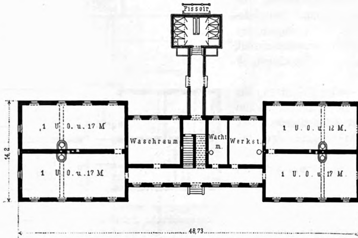
Mannschafts-Wohngebäude für 1 Eskadron. — Erdgeschofs 143) .
