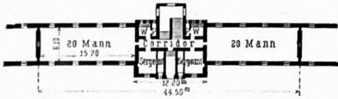
System der Garde-Infanteriekaserne zu Chelsea.
