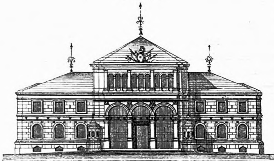
Ansicht.
