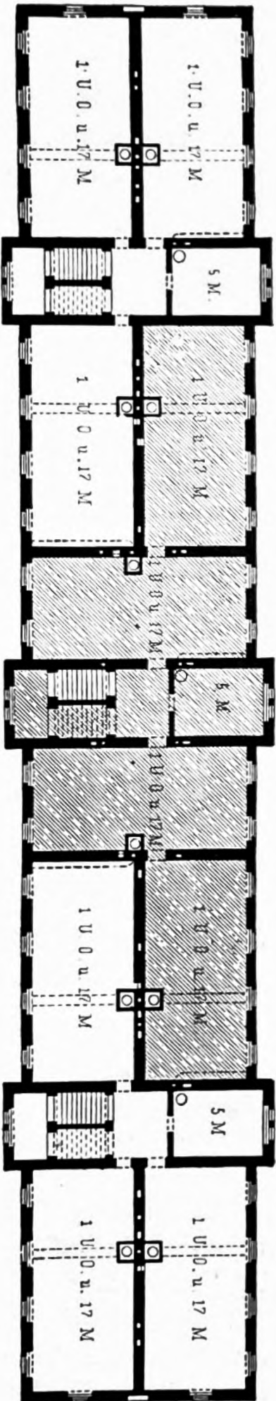
I. Ober- geschofs.
