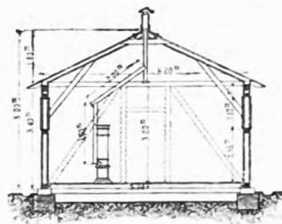
Hölzerne Mannschaftsbaracke.
