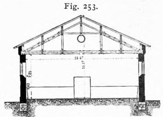
Querschnitt eines älteren Reithauses. 1/500 w. Gr.
