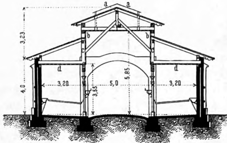
Neueres sächsisches Stallgebäude.
