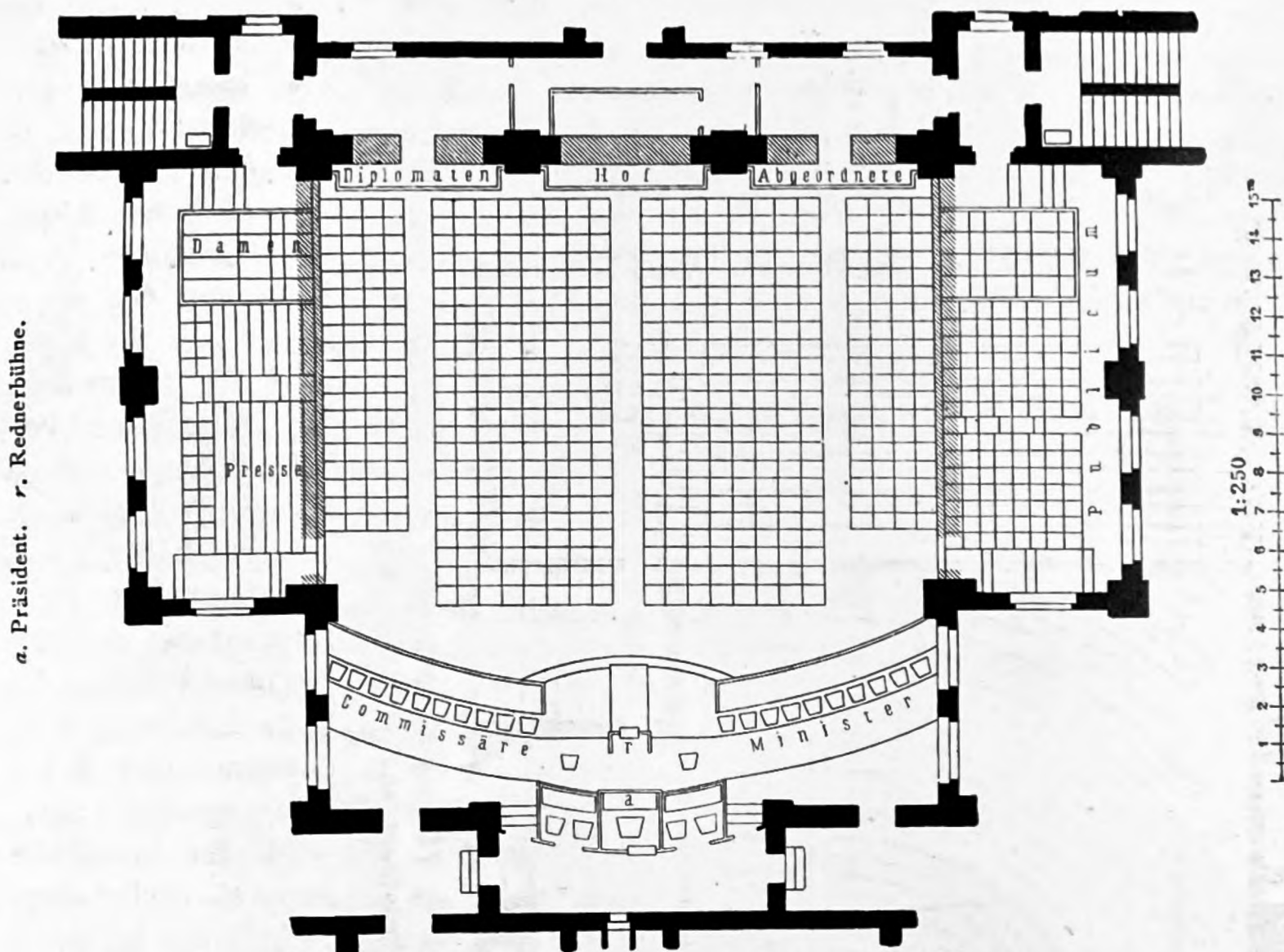
Sitzungssaal des früheren Herrenhauses zu Berlin.
