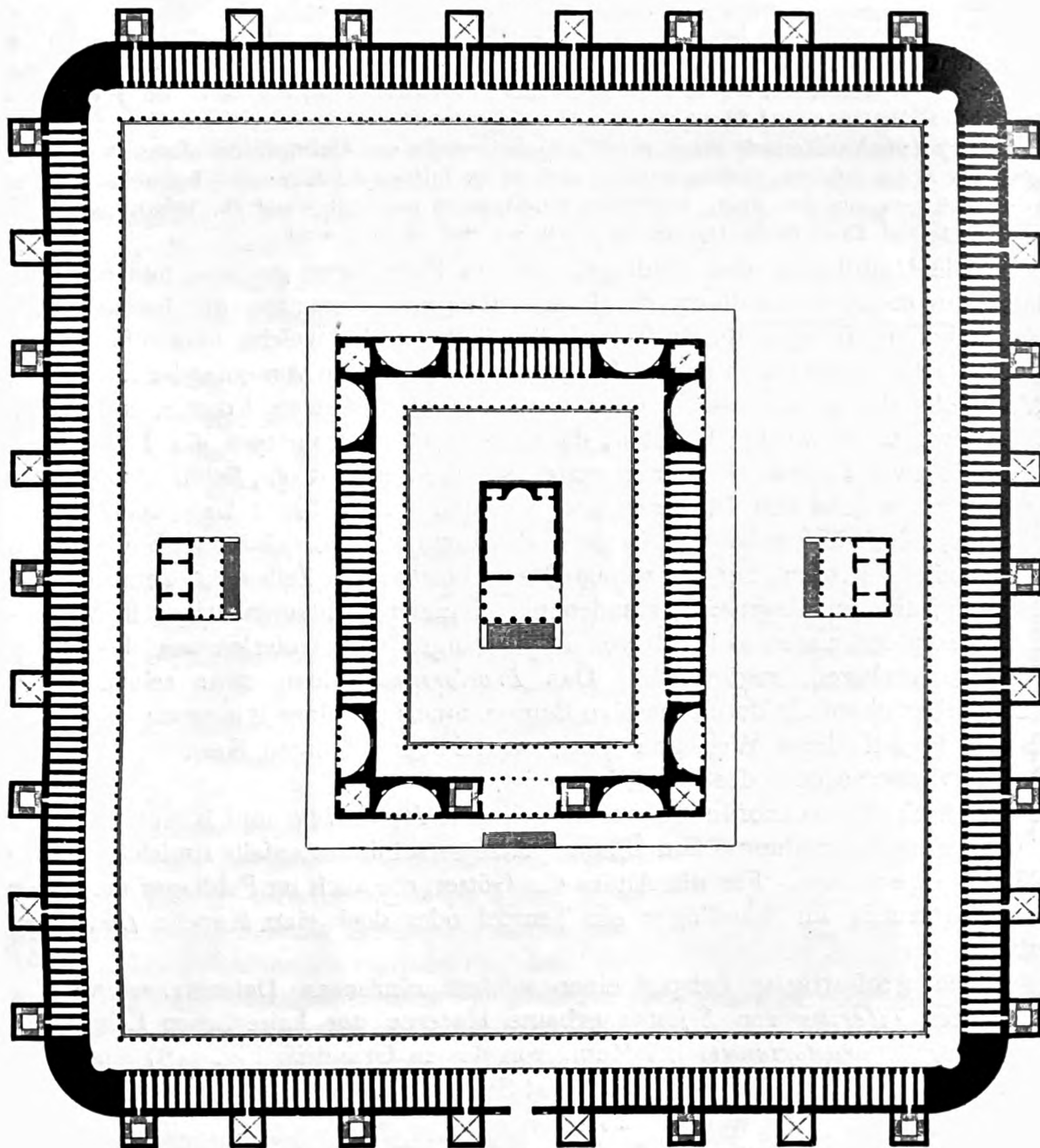
Castrum praetorianum bei Rom 91) . — \frac{1}{3000} w. Gr.
