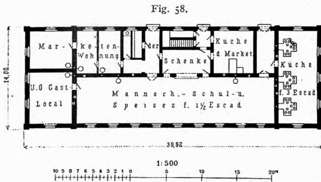
Marketenderei- und Küchengebäude einer österreichischen Kavallerieregiments-Kaserne 103) .
