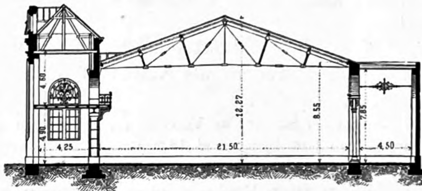
Querschnitt.
