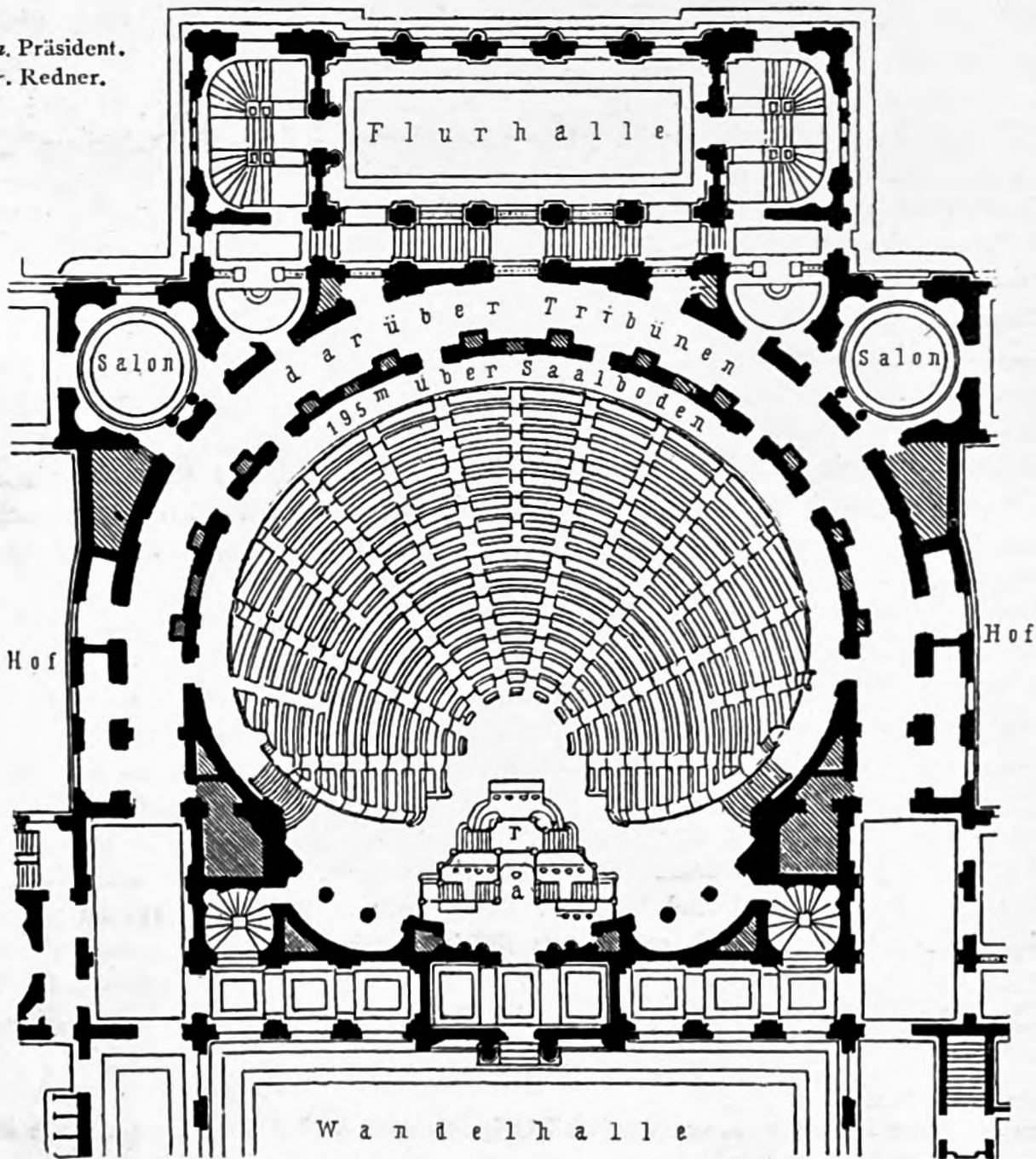
De Joly's Entwurf zu einem Sitzungssaale der Deputiertenkammer zu Paris 26) .
