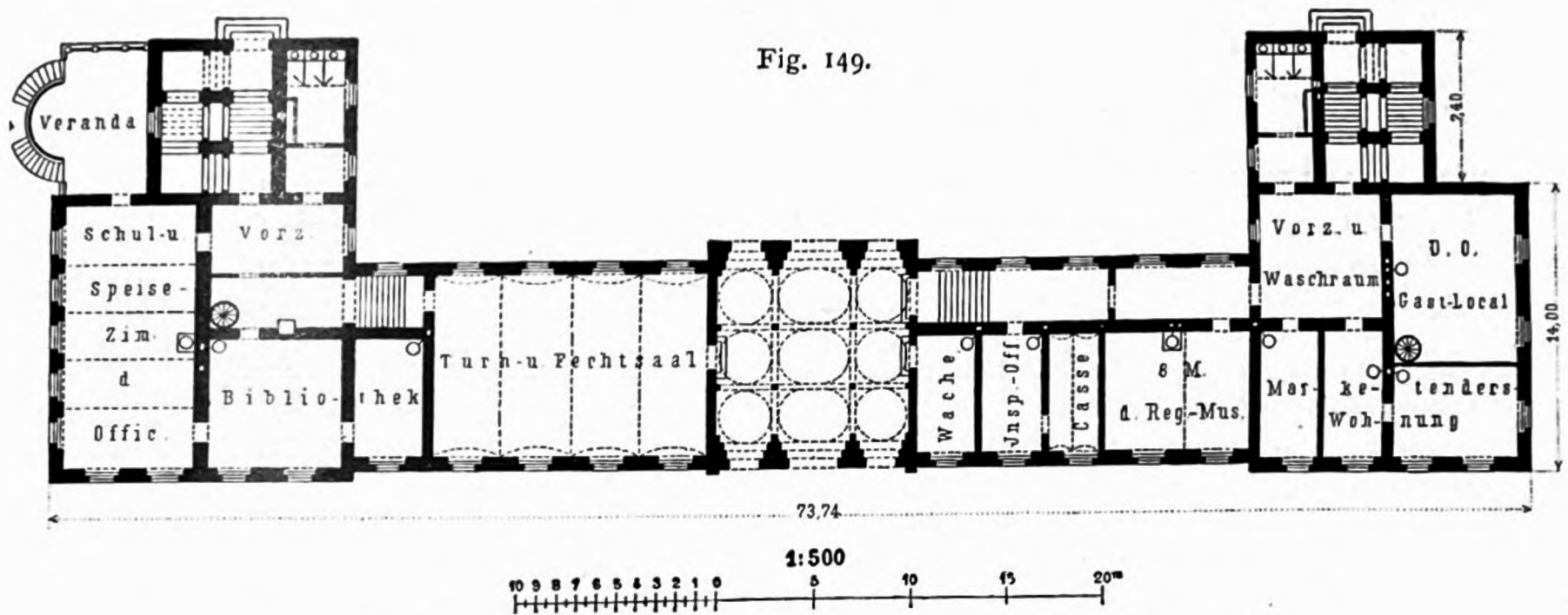
Stabsgebäude für eine österreichische Infanterieregiments-Kaserne 139) .
