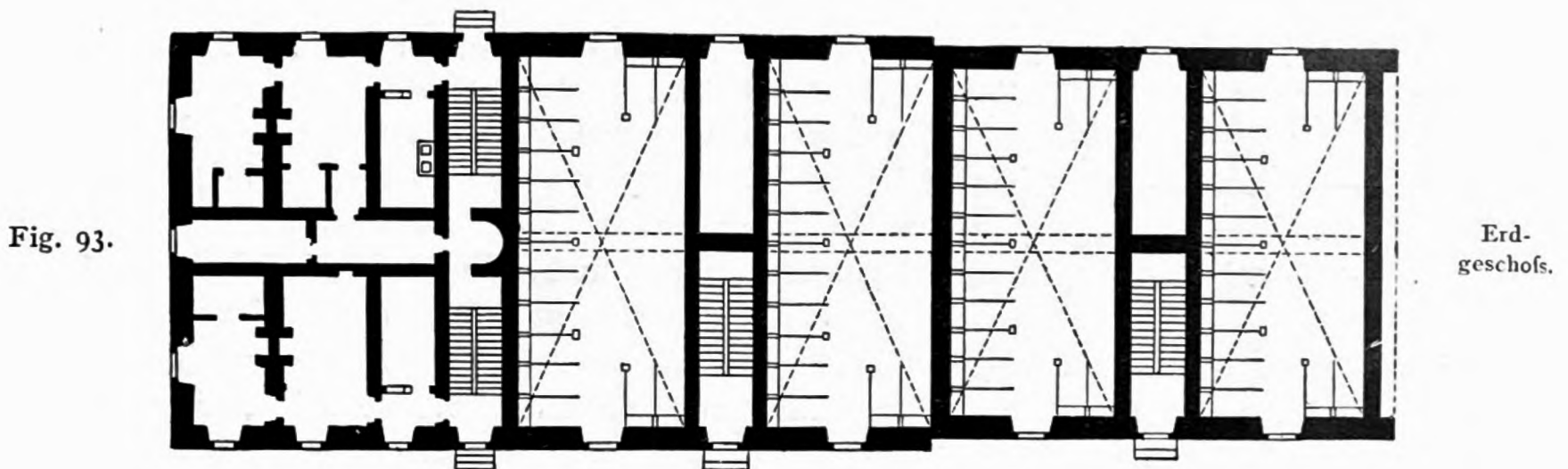
Kavalleriekaserne Chambières zu Metz 128) .
