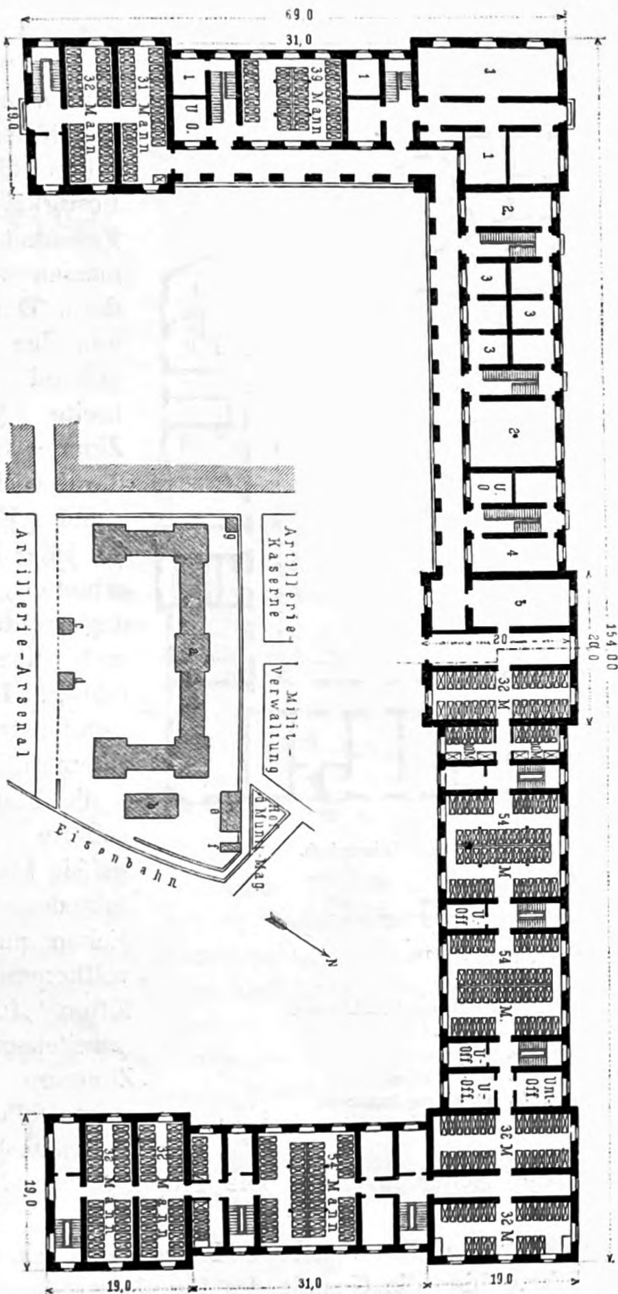
Fig. 104. Erdgeschoss. 1. Magazine. 2. Stallungen. 3. Wohnungen der Werkstättenmeister. 4. Rapportzimmer. 5. Tanzsaal.
