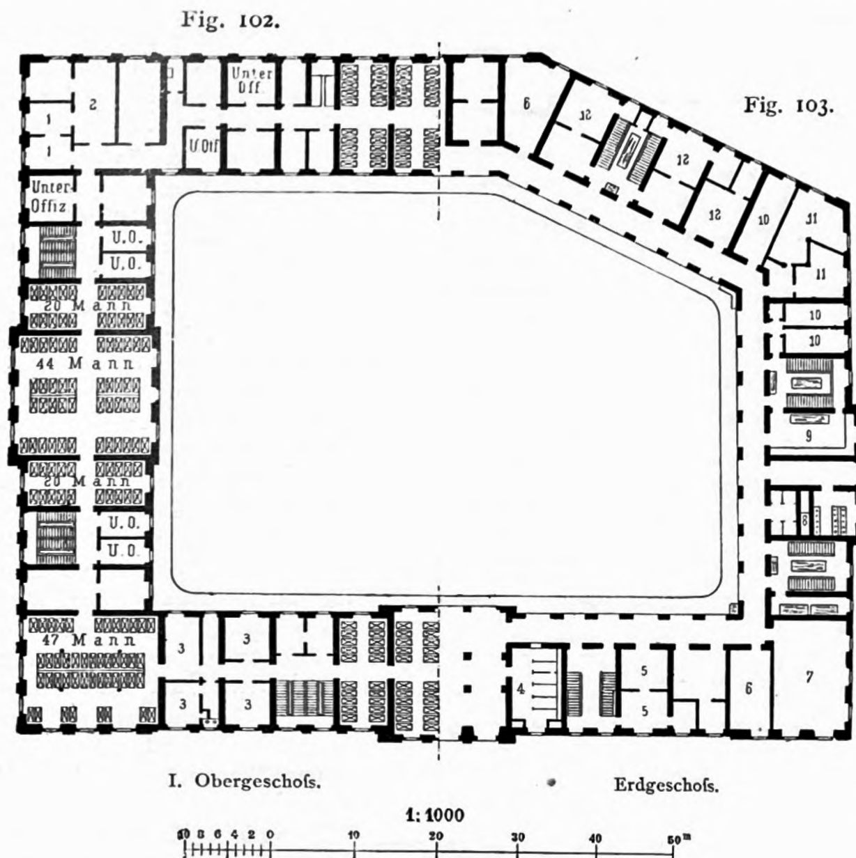
Napoleons-Kaserne zu Paris 132) .
