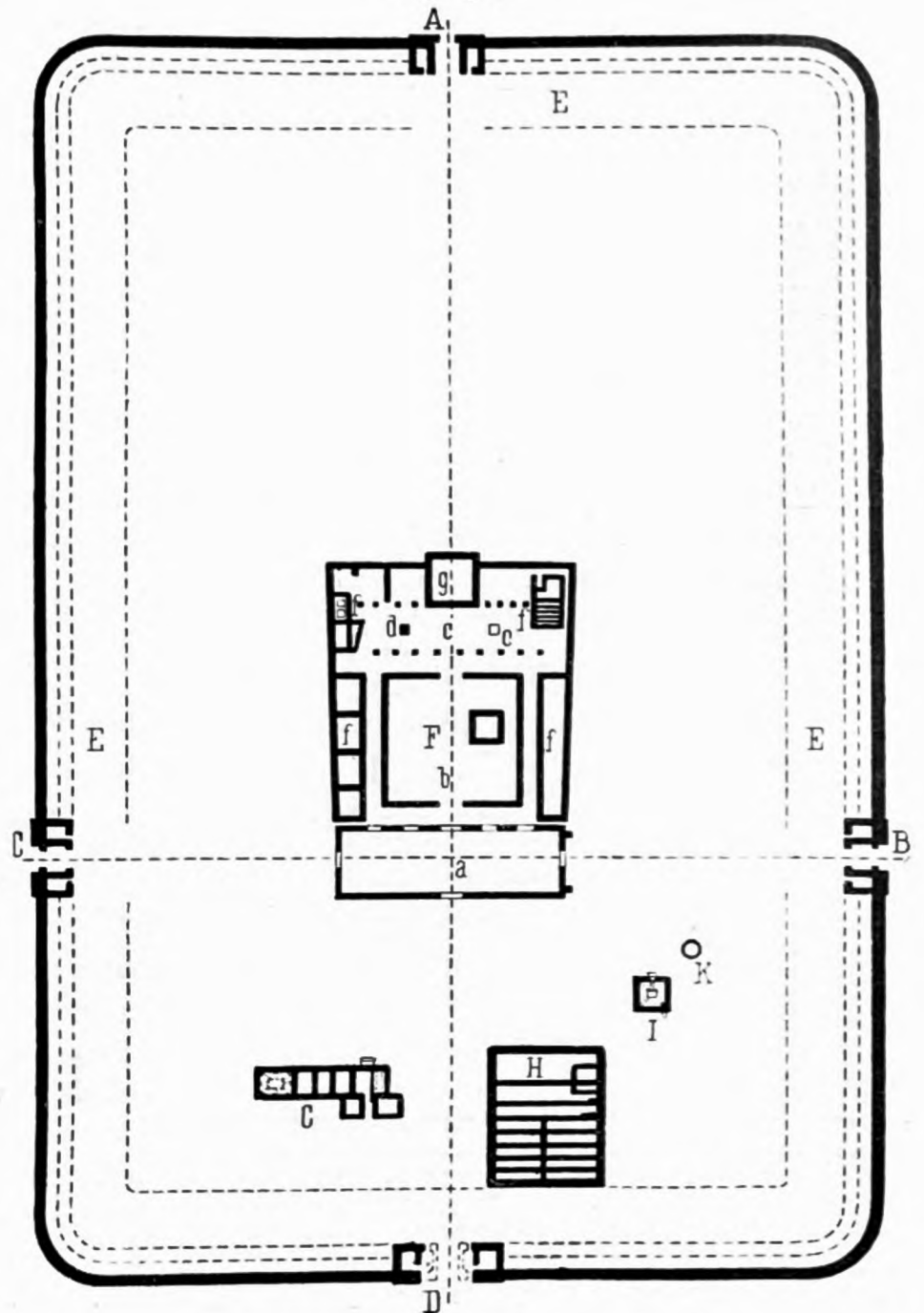
Römisches Kastell bei Homburg 95) .
