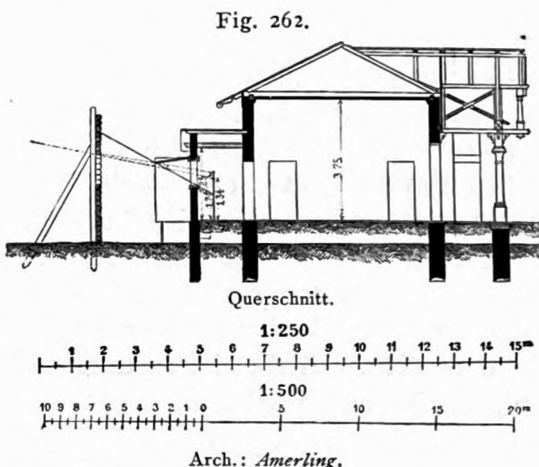
Schießhaus mit zwei Schießständen.
