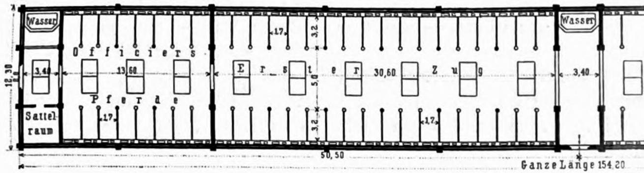
Eskadronstallung zu Dresden.
