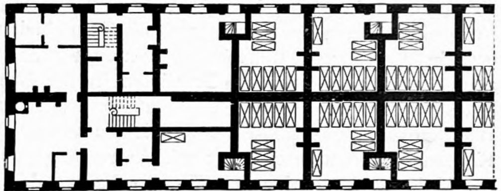
Infanteriekaserne zu Hâvre 128) .
