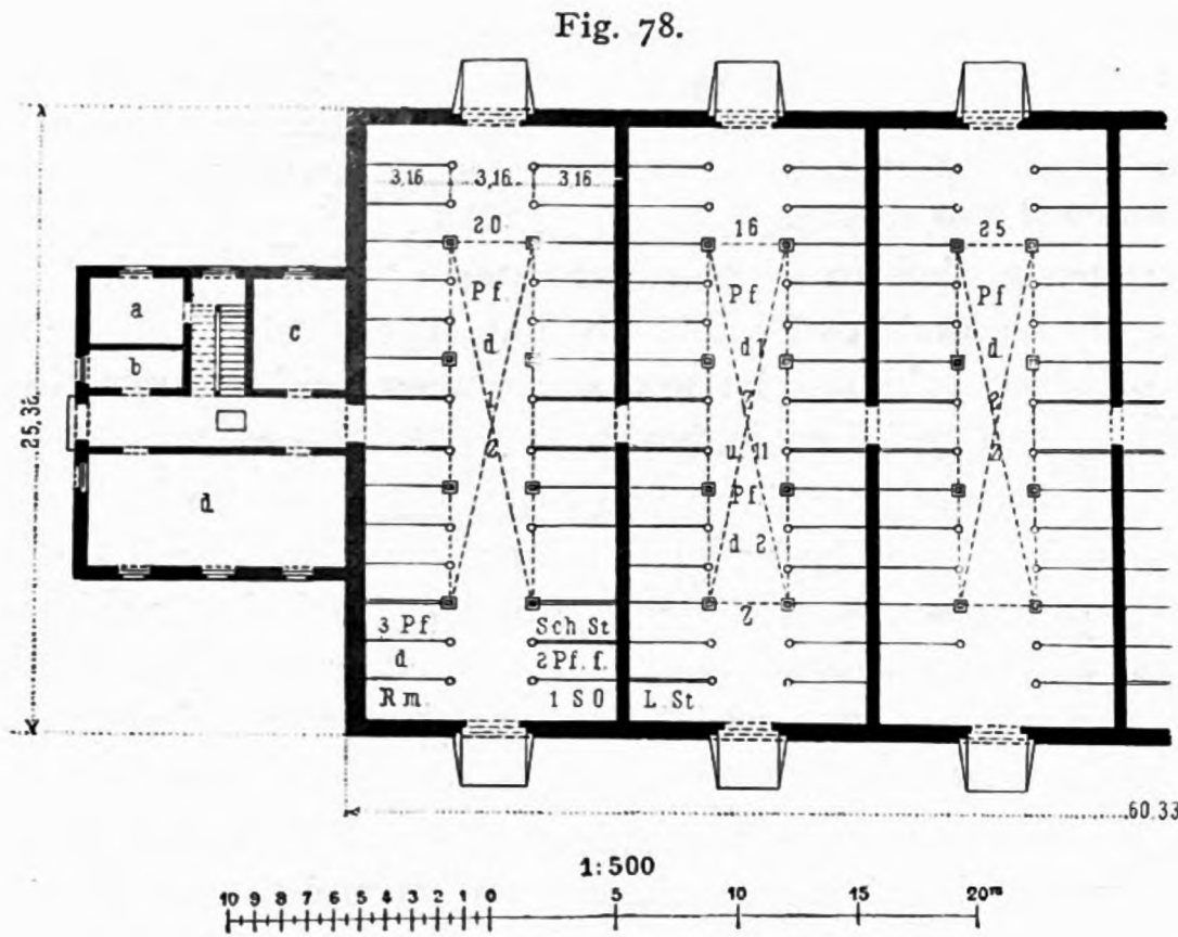
Österreichische Eskadronstallung 120) .
