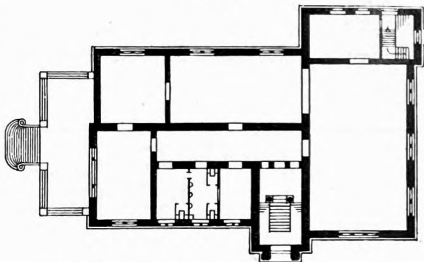
Offiziers-Speiseanstalt des 2. Eisenbahnregiments zu Berlin. 1/500 w. Gr.
