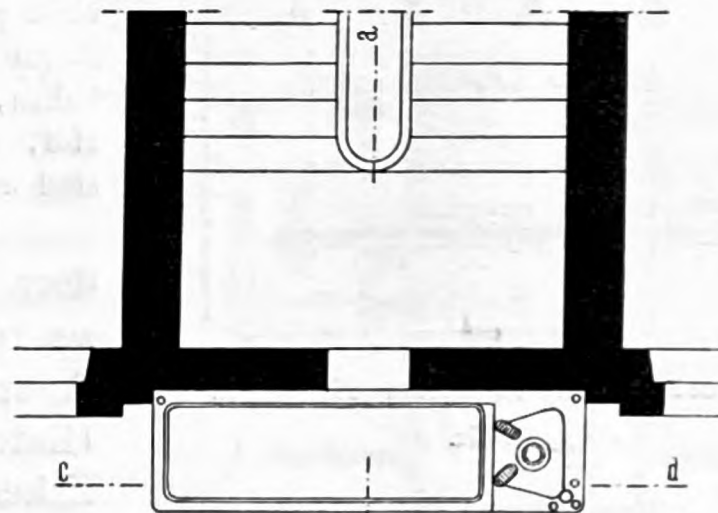
Grundriß.
