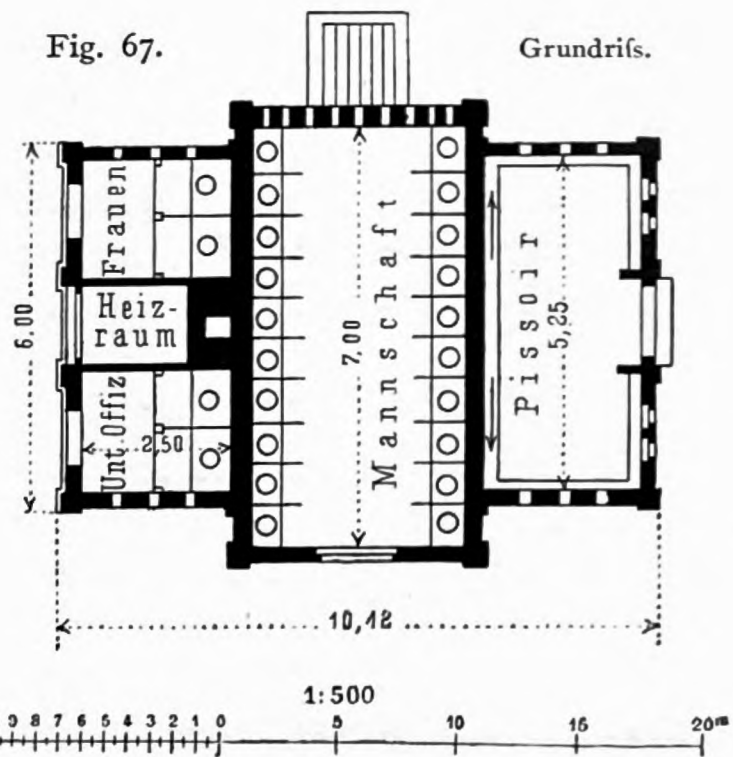
Abortgebäude für ein Bataillon in preussischen Kasernen.
