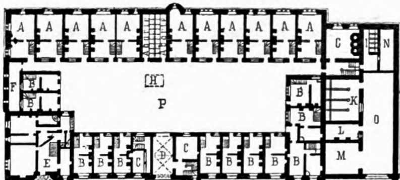
Milizkaserne zu Chester. — \frac{1}{1000} w. Gr.
