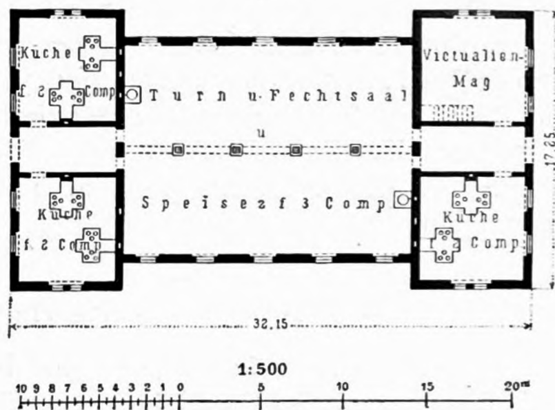
Turn-, Fechtsaal- und Küchengebäude für ein österreichisches Infanterieregiment 110) .
