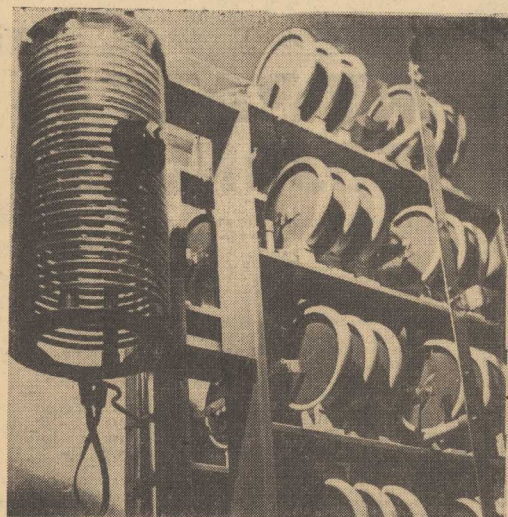
Bateria kondensatorów
