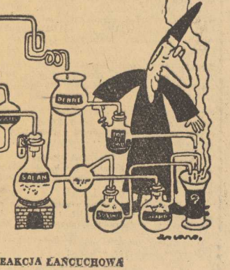
REAKCJA ŁANUCHOWA
