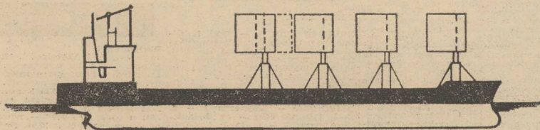
Szybetka masowca B-545 z pednikiem wiatrowym
