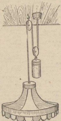
Sposób wykonania opuszczanej lampy.
