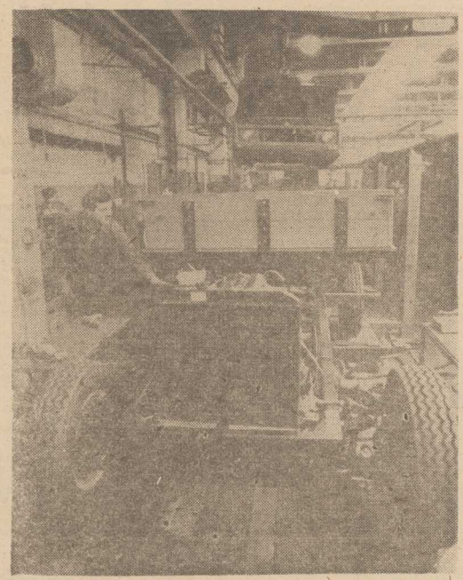
W FABRYCE Samochodów Rolniczych w Poznaniu trwa montaż „Tarpana 237”. Ten najnowszy model posiada ładowność 1 tony i nowoczesny układ nadwozia. Produkowany jest w 5 wersjach. W ubiegłym roku zmontowano w poznańskiej fabryce 4250 sztuk pojazdów, a w tym przewiduje się dostarczenie 4800 samochodów. NA ZDJĘCIU: montaż „Tarpana 237”. (CAF — R. Królak)
