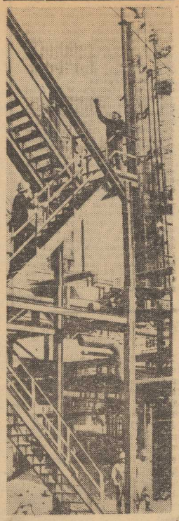
BASZKIRIA (RFSRR). W Nowo-Ufimskich zakładach przeróbki ropy naftowej buduje się obecnie specjalne urządzenie do rafinacji olejów napędowych i produkcji wysokogatunkowej benzyny, nie zawierającej związków siarki. Skomplikowana aparatura ma dużą wydajność, zajmuje zaś stosunkowo niewielką przestrzeń. Na zdjęciu: montaż nowej rafinerii. (CAF — TASS)
