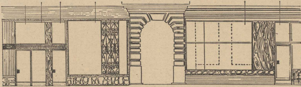
FRAGMENT elewacji zaprojektowanej dla modernizowanych obecnie sklepów przy al. Wojska Polskiego.
