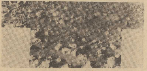
ZDJĘCIE kamienistej powierzchni Marsa wykonane przez sondę kosmiczną „Viking-2”
