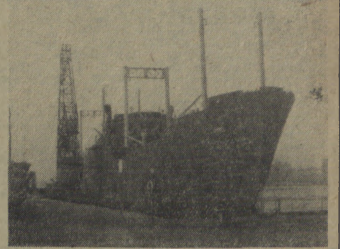
Ostatnio w Stoczni Gdańskiej został spuszczonej na wodę statek pełnomorski typu węglowie. Jest to setny statek zbudowany po wojnie przez polski przemysł okrętowy. Statek ten został wykonany pzedterminowo przez załogę Stoczni Gdańskiej, w ramach zobowiązań dla uczczenia II Zjazdu PZPR. Na zdjęciu: setny statek w kanale wyposażeniowym w Stoczni Gdańskiej. (Fot. CAF)
