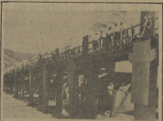
W ramach wielkich robót irygacyjnych w Chińskiej Republice Ludowej wybudowany został wielki basen na rzece Jang-tse, dzięki któremu 3-milionowa ludność Kienghan w prowincji Hupeh, wyzwoliła się od klęski powodzi, którymi była nękana od 1000 lat. Na zdjęciu: tama w Huangantou, której długość wynosi 337 m.
